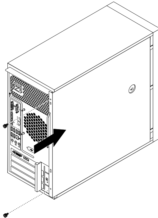
Abbildung 70. Serverabdeckung wieder installieren
