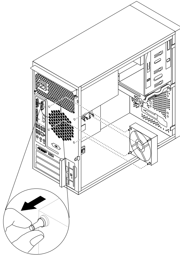
Abbildung 64. Lüftungsbaugruppe an der Rückseite installieren
