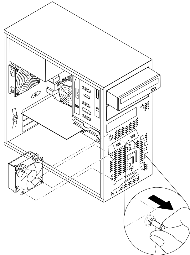
Abbildung 62. Lüftungsbaugruppe an der Vorderseite installieren
