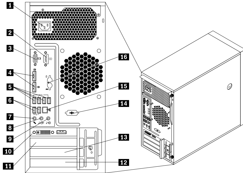
Abbildung 4. Positionen der Anschlüsse an der Rückseite
