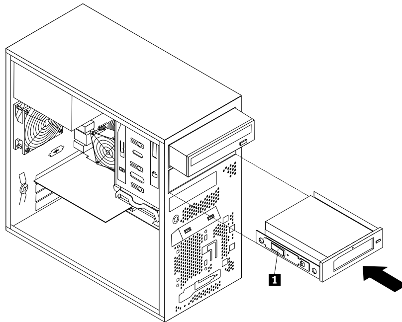
Abbildung 54. RDX-Laufwerk installieren
