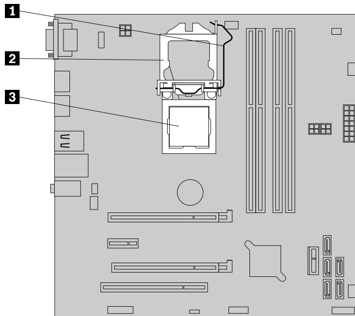
Abbildung 65. Zugriff auf den Mikroprozessor
