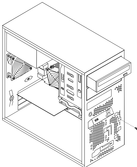
Abbildung 60. Audio- und USB-Baugruppe an der Vorderseite entfernen
