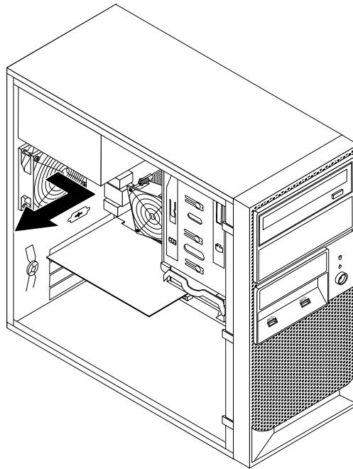
Abbildung 63. Lüftungsbaugruppe an der Rückseite entfernen
