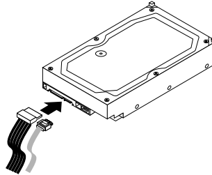
Abbildung 24. SATA-Festplattenlaufwerk anschließen
