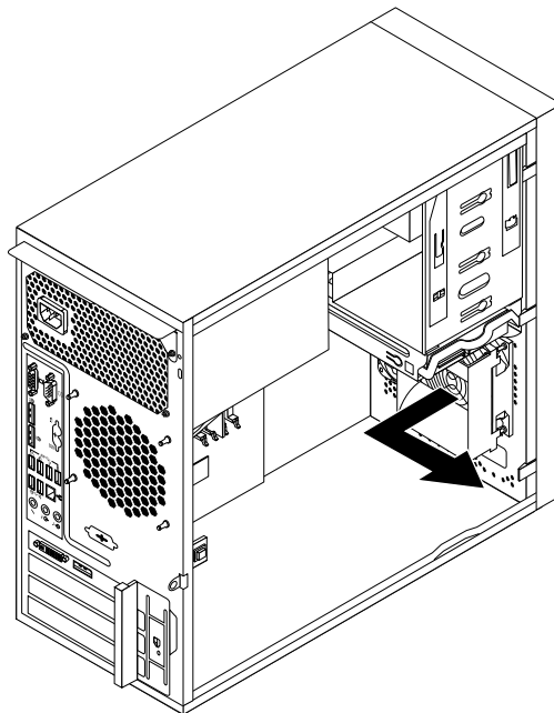
Abbildung 61. Lüftungsbaugruppe an der Vorderseite entfernen
