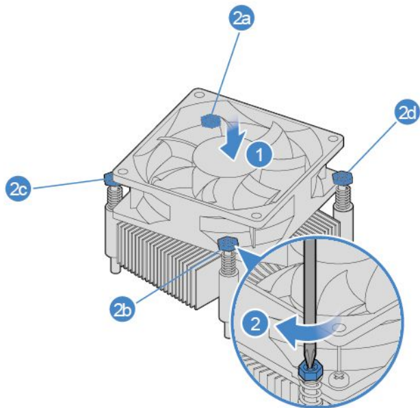
図 28. ヒートシンクおよびファンの取り付け
