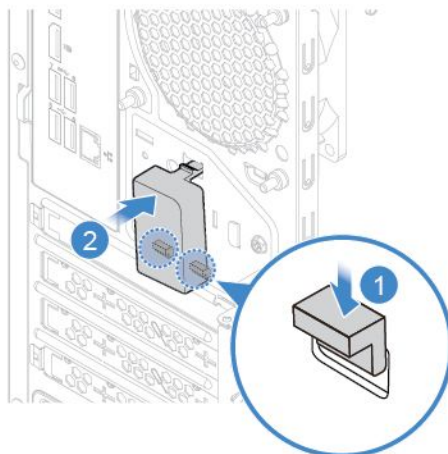
図70. 背面 Wi-Fi アンテナ・カバーの取り付け
