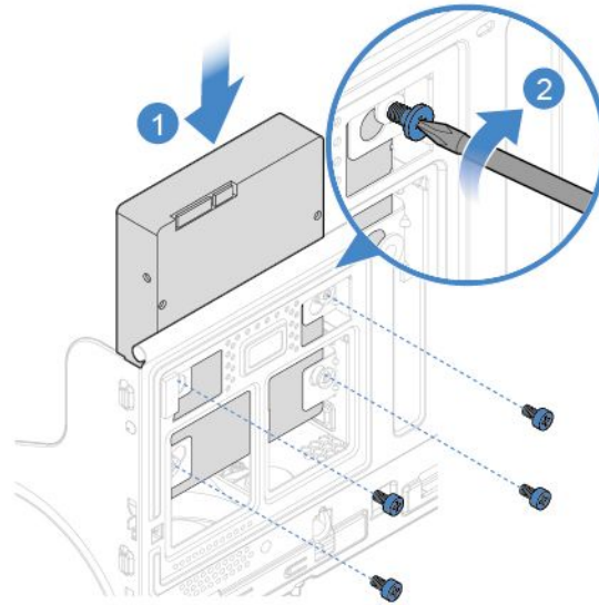
図 18. 3.5 型プライマリー・ストレージ・ドライブの取り付け
