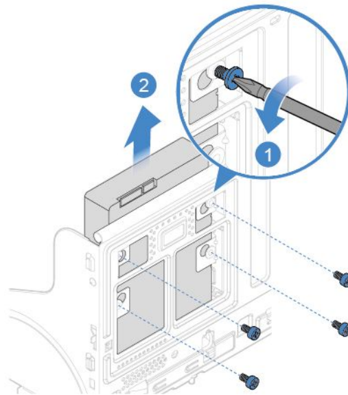
図 17. 3.5 型プライマリー・ストレージ・ドライブの取り外し
