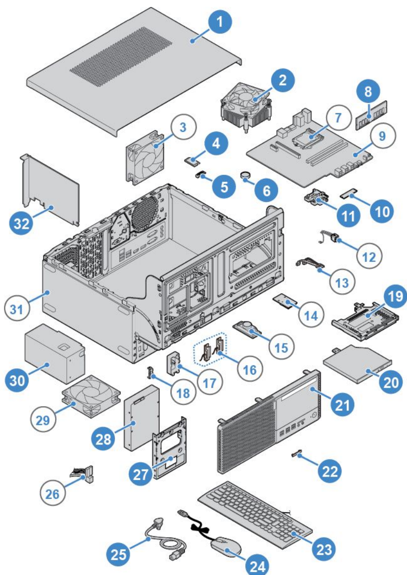
図7. FRU (CRU を含む) の位置
