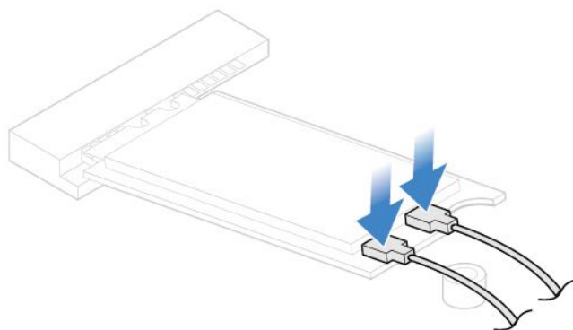
図45. Wi-Fi アンテナ・ケーブルの接続
