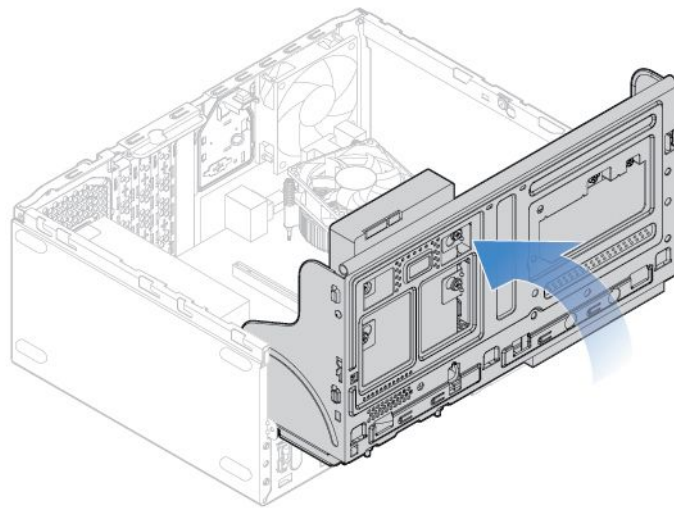
図 16. ドライブ・ベイを下方に回す
