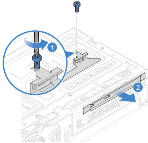
図13. 光学式ドライブ・ブラケットの取り外し
