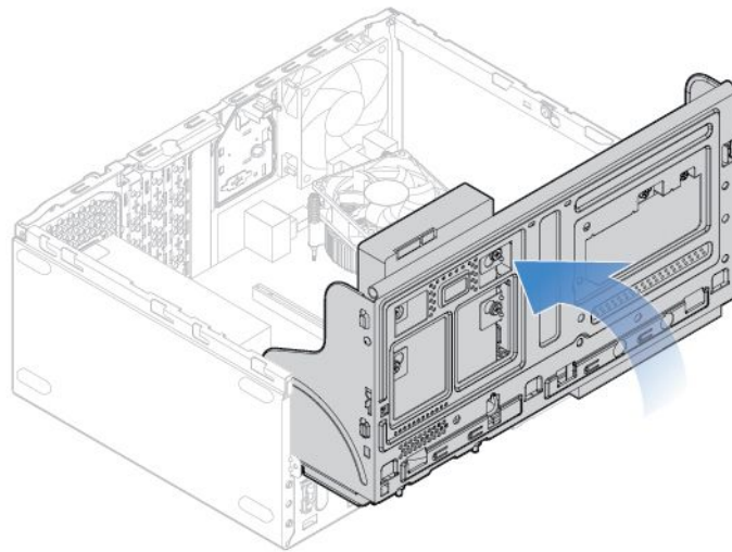
図 75. ドライブ・ベイを下方に回す
