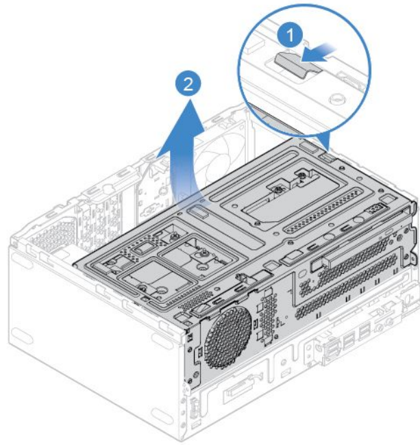
図 72. ドライブ・ベイを上方に持ち上げる
