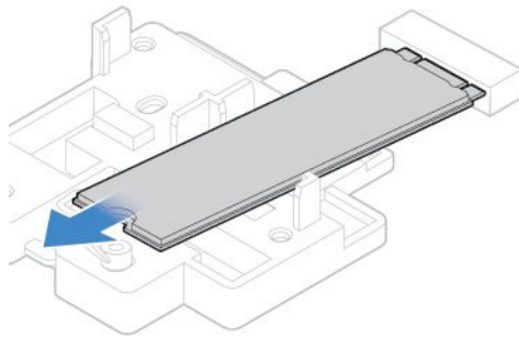
図 48. M.2 ソリッド・ステート・ドライブの取り外し
