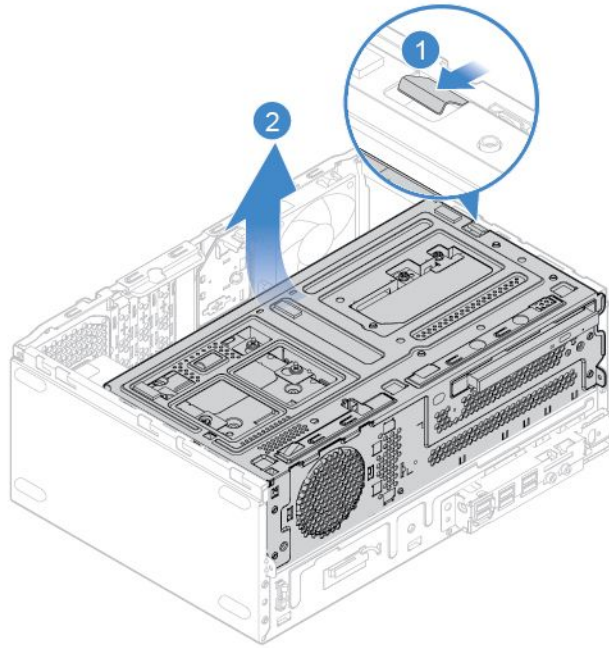
図 15. ドライブ・ベイを上方に持ち上げる
