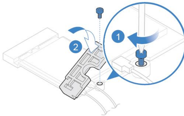
図 40. Wi-Fi カード・シールドの取り付け
