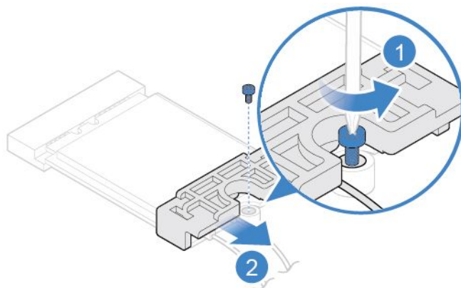
図35. Wi-Fi カード・シールドの取り外し
