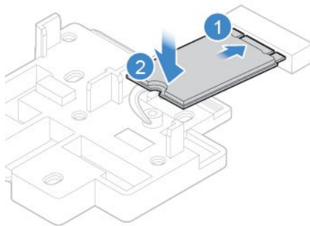
図52. M.2 ソリッド・ステート・ドライブの取り外し
