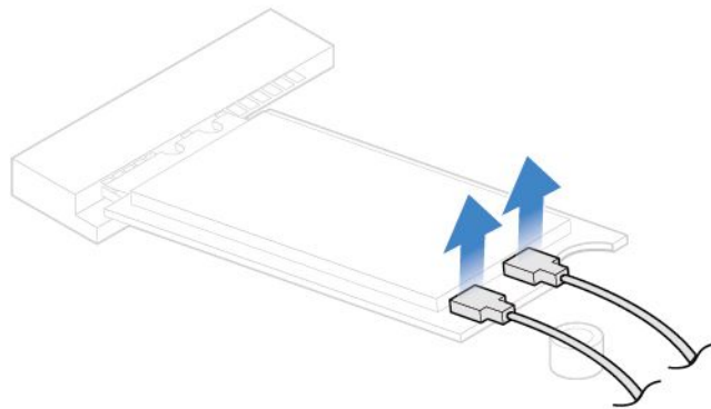
図 42. Wi-Fi アンテナ・ケーブルの取り外し
