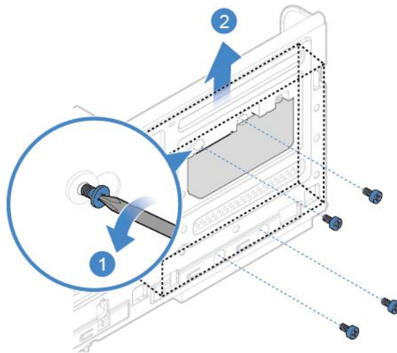
図 19. 3.5 型セカンダリー・ストレージ・ドライブの取り外し
