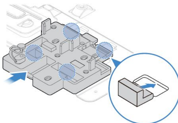
図 56. M.2 ソリッド・ステート・ドライブ・ブラケットの取り付け
