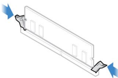
図26. メモリー・モジュールをラッチで固定する
