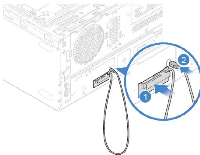
図 66. 前面 Wi-Fi アンテナの取り付け
