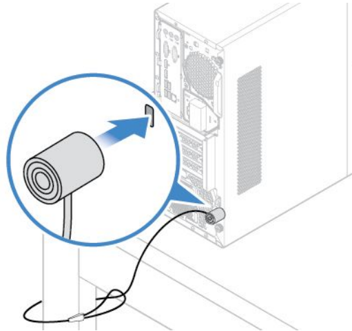
図 6. Kensington スタイルのケーブル・ロックの取り付け
