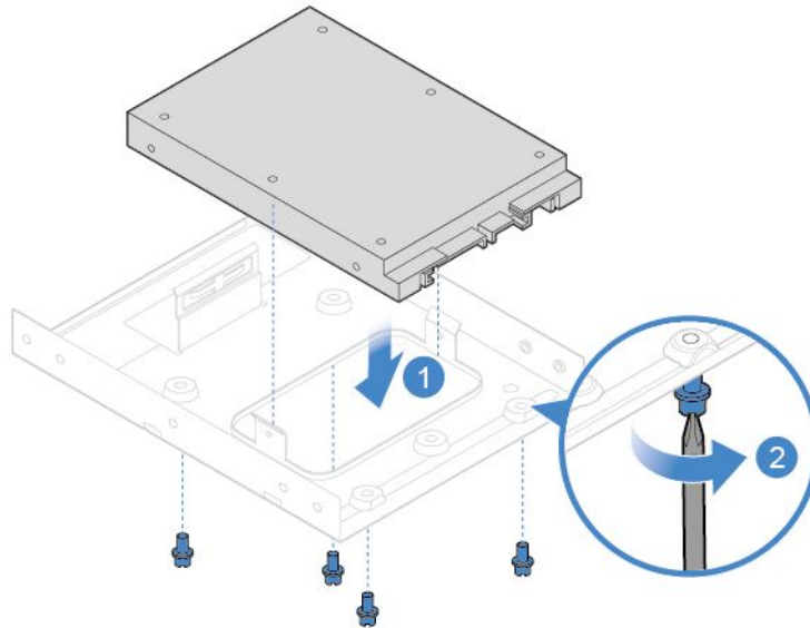
図22. 2.5 型ストレージ・ドライブのストレージ・コンバーターへの取り付け
