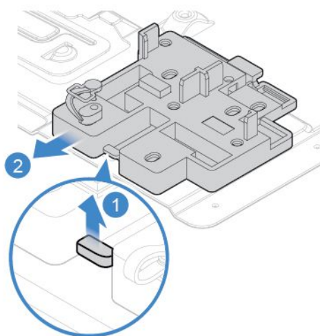
図 55. M.2 ソリッド・ステート・ドライブ・ブラケットの取り外し
