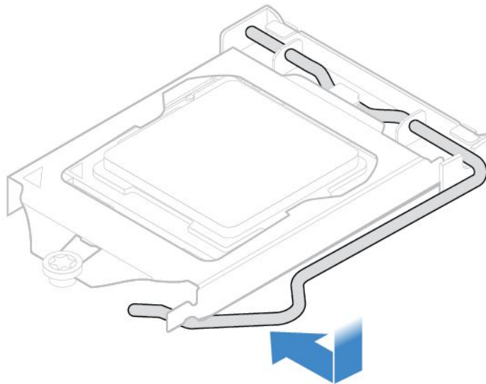
図 85. ハンドルを使用して、固定具を固定する
