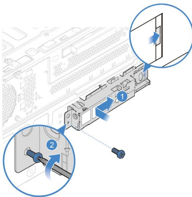
図 79. 前面 I/O ブラケットの取り付け
