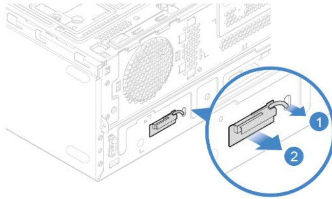
図 65. 前面 Wi-Fi アンテナの取り外し
