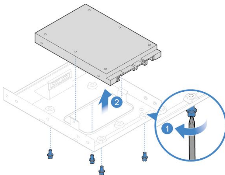
図21. 2.5 型ストレージ・ドライブのストレージ・コンバーターからの取り外し
