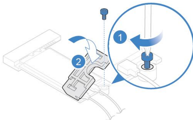
図46. Wi-Fi カード・シールドの取り付け
