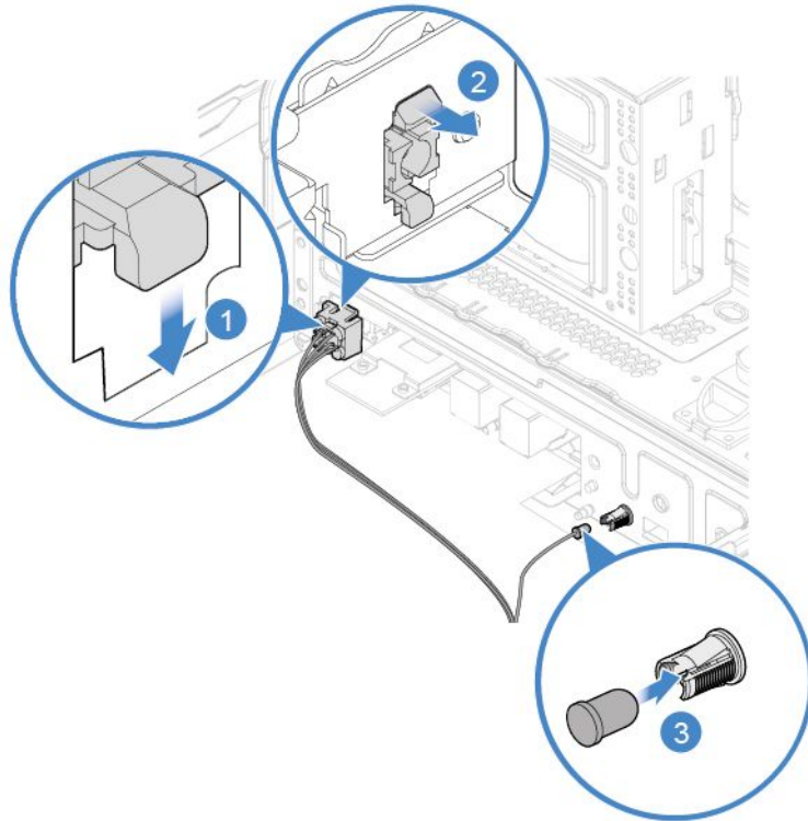
図 74. 電源ボタン・ボードの取り付け
