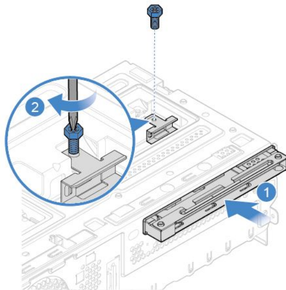
図14. 光学式ドライブ・ブラケットの取り付け
