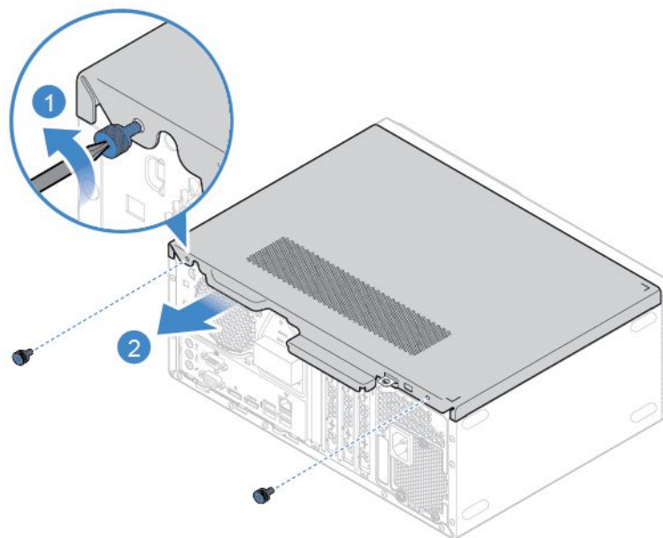
図8. コンピューター・カバーの取り外し
