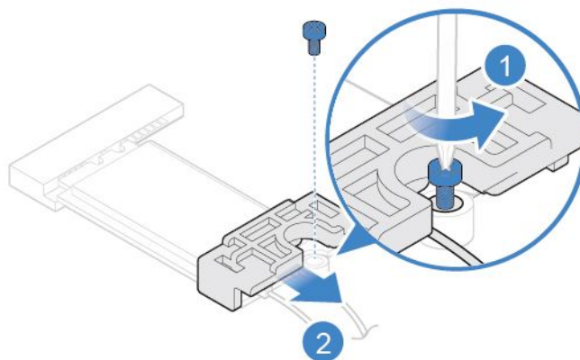
図 41. Wi-Fi カード・シールドの取り外し
