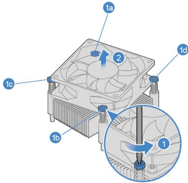
図 27. ヒートシンクおよびファンの取り外し
