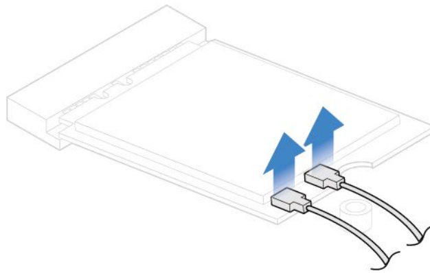
図 36. Wi-Fi アンテナ・ケーブルの取り外し
