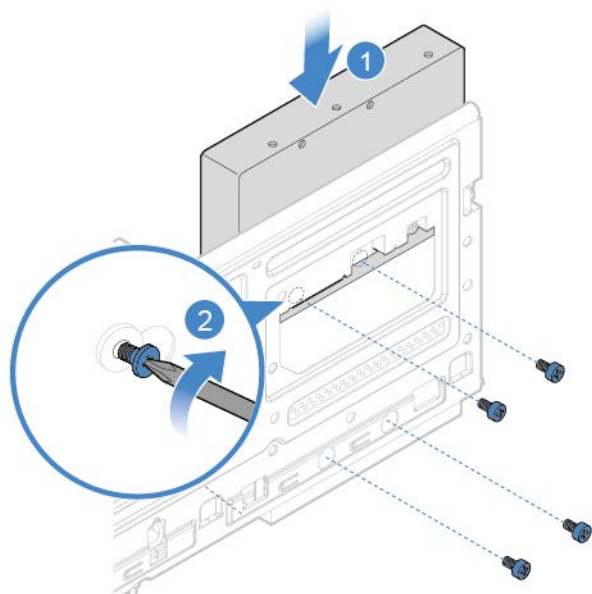
図20. 3.5 型セカンダリー・ストレージ・ドライブの取り付け
