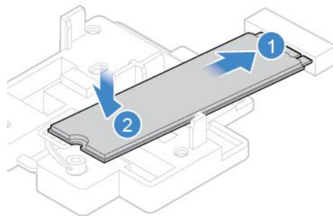
図 49. M.2 ソリッド・ステート・ドライブの取り付け
