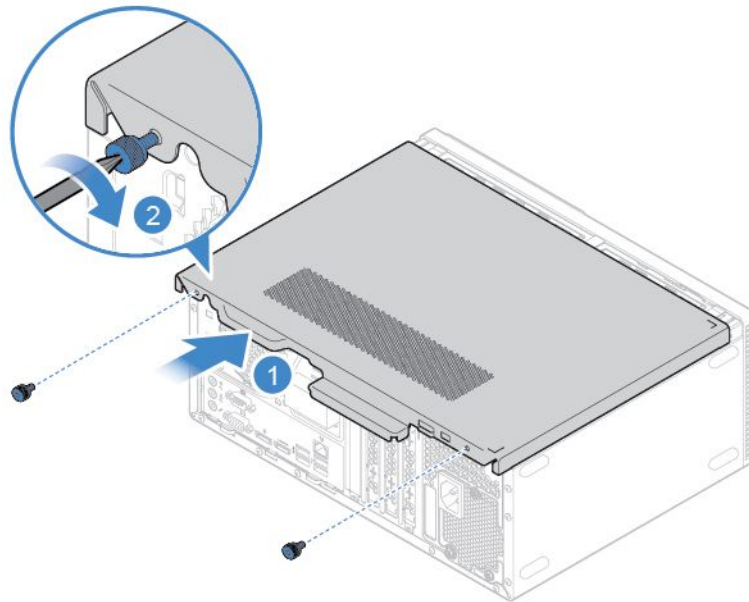
図88. コンピューターのカバーを元の位置に戻す
