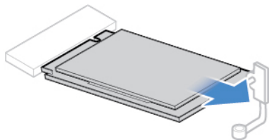
Figura 21. Removendo a unidade de estado sólido M.2
