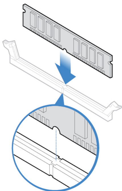
Figura 29. Removendo um Módulo de Memória
