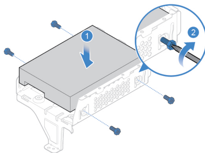
Figura 10. Instalando a unidade de armazenamento de 3,5 polegadas
