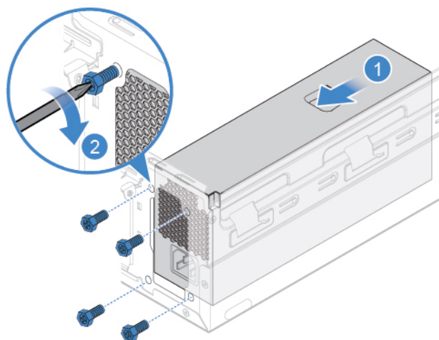
Figura 36. Instalando o conjunto da fonte de alimentação
