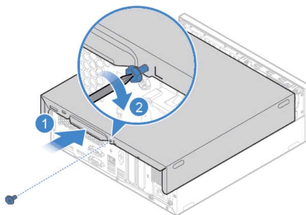
Figura 37. Reinstalando a tampa do computador
