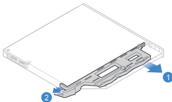
Figura 5. Removendo o suporte da unidade óptica
