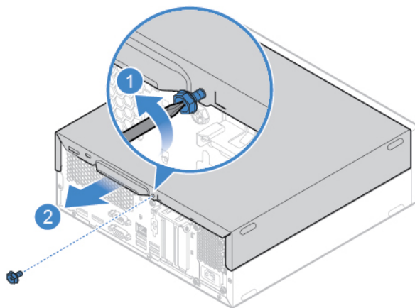
Figura 1. Removendo a tampa do computador
