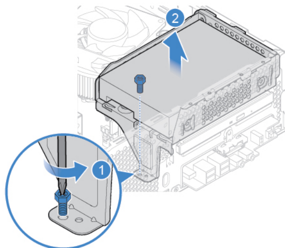
Figura 8. Removendo o suporte da unidade de armazenamento
