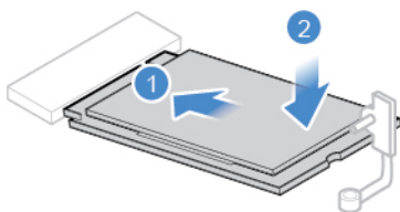
Figura 22. Instalando a unidade de estado sólido M.2
