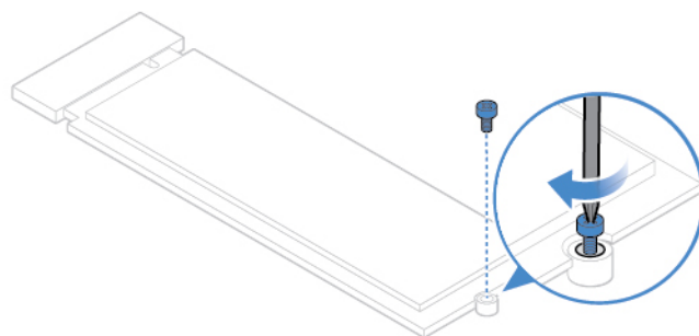
Figura 18. Instalando a unidade de estado sólido M.2
