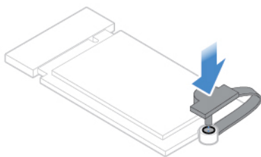
Figura 22. Instalando a unidade de estado sólido M.2
