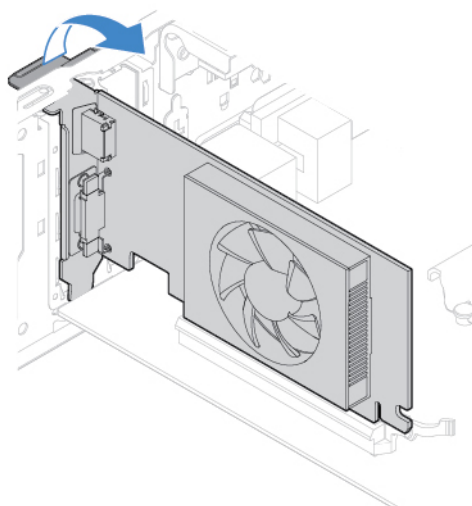
Figura 34. Prendendo uma placa PCI Express com a trava
