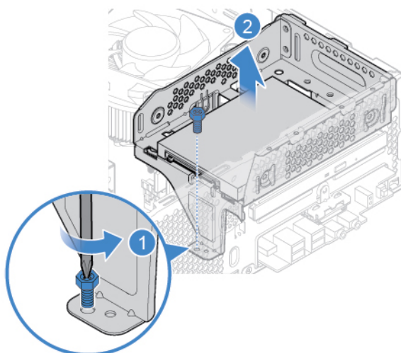
Figura 12. Removendo o suporte da unidade de armazenamento
