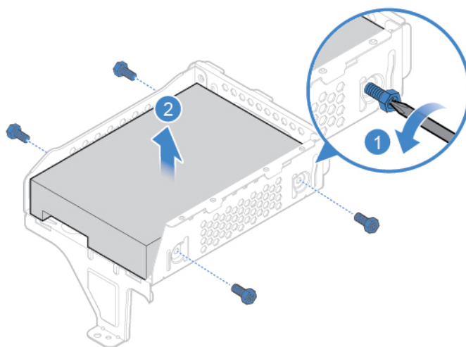
Figura 9. Remova a unidade de armazenamento de 3,5 polegadas
