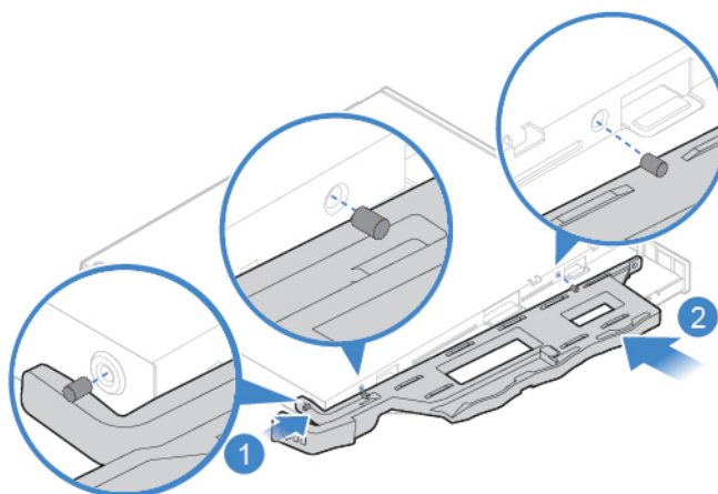
Figura 6. Instalando o suporte da unidade óptica
