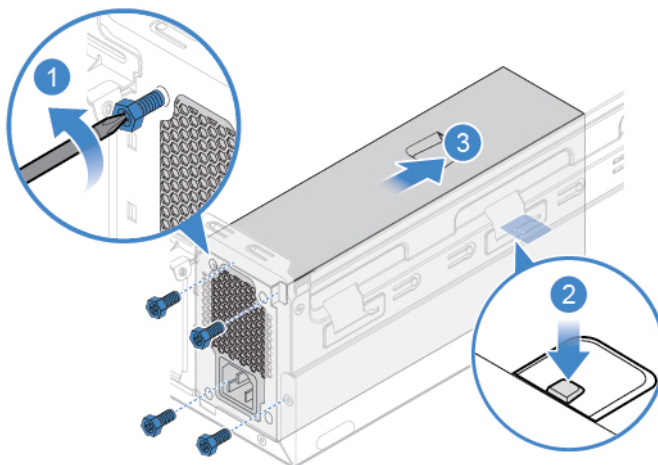
Figura 35. Removendo a montagem da fonte de alimentação
