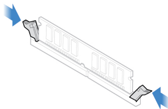
Figura 31. Prendendo um módulo de memória com as travas
