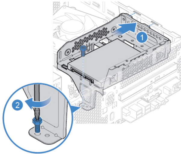
Figura 15. Instalando o suporte da unidade de armazenamento
