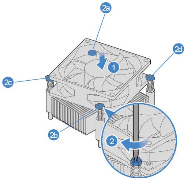
図 12. ヒートシンクおよびファンの取り付け
