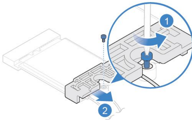
図29. Wi-Fi カード・シールドの取り外し
