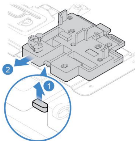
図49. M.2 ソリッド・ステート・ドライブ・ブラケットの取り外し
