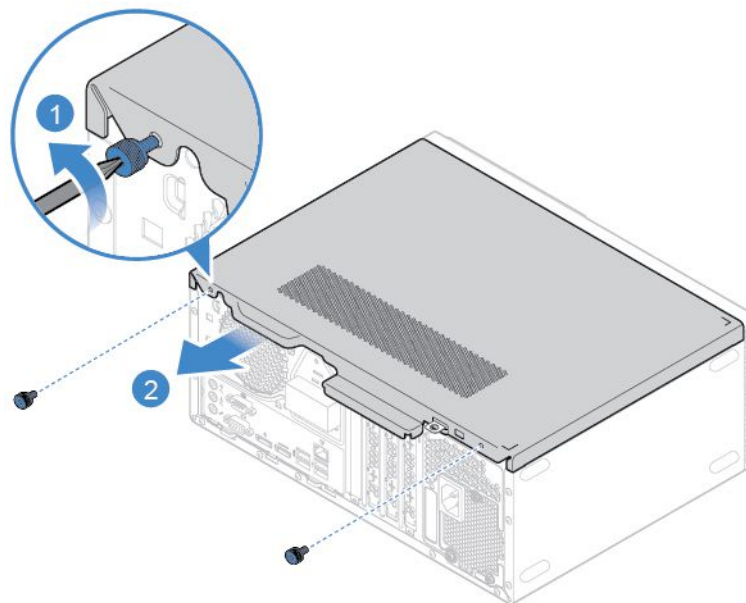
図1. コンピューター・カバーの取り外し
