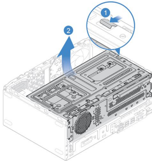
図9. ドライブ・ベイを上方に持ち上げる
