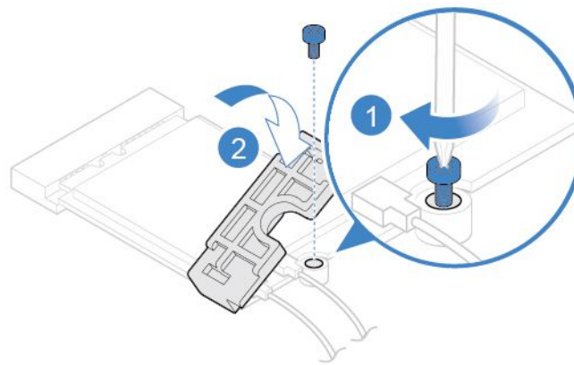
図 34. Wi-Fi カード・シールドの取り付け
