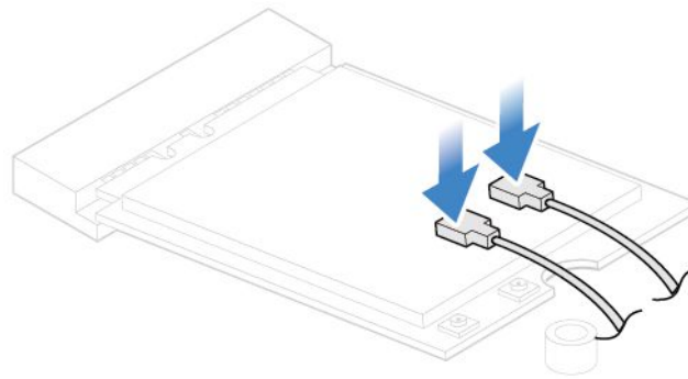
図 33. Wi-Fi アンテナ・ケーブルの接続
