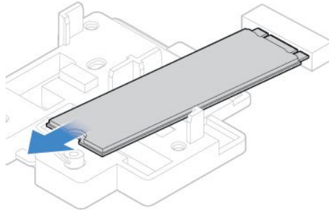
図42. M.2 ソリッド・ステート・ドライブの取り外し
