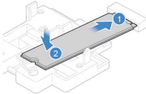
図43. M.2 ソリッド・ステート・ドライブの取り付け
