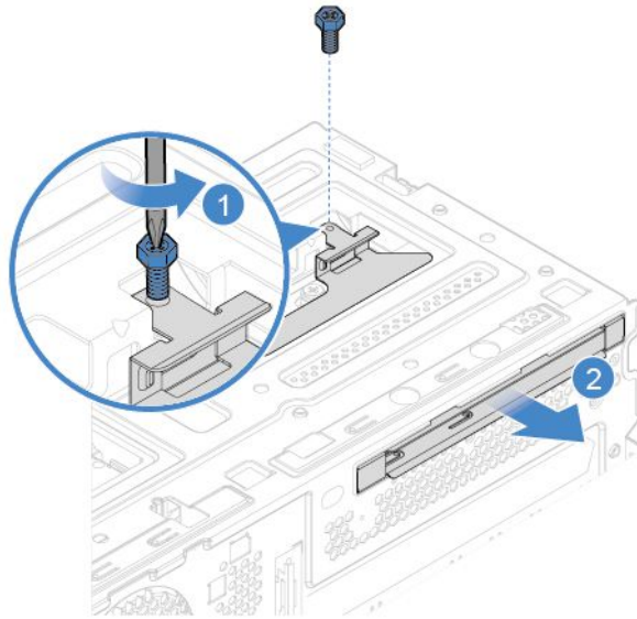
図7. 光学式ドライブ・ブラケットの取り外し
