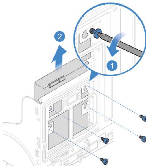
図 13. 3.5 型プライマリー・ストレージ・ドライブの取り外し
