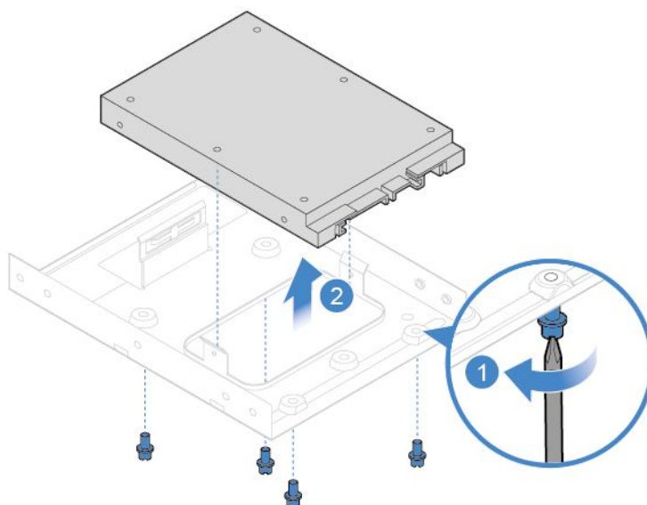
図 17. 2.5 型ストレージ・ドライブのストレージ・コンバーターからの取り外し
