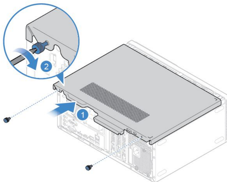
図2. コンピューターのカバーを元の位置に戻す
