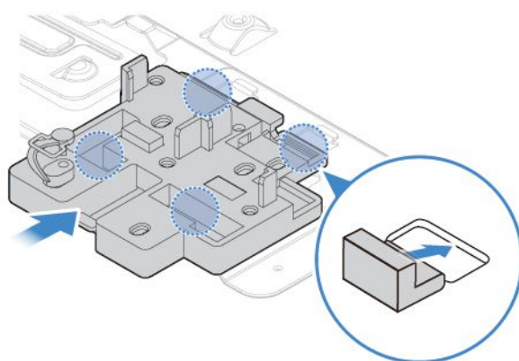
図50. M.2 ソリッド・ステート・ドライブ・ブラケットの取り付け
