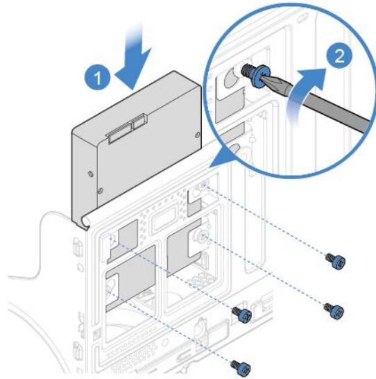
図 14. 3.5 型プライマリー・ストレージ・ドライブの取り付け
