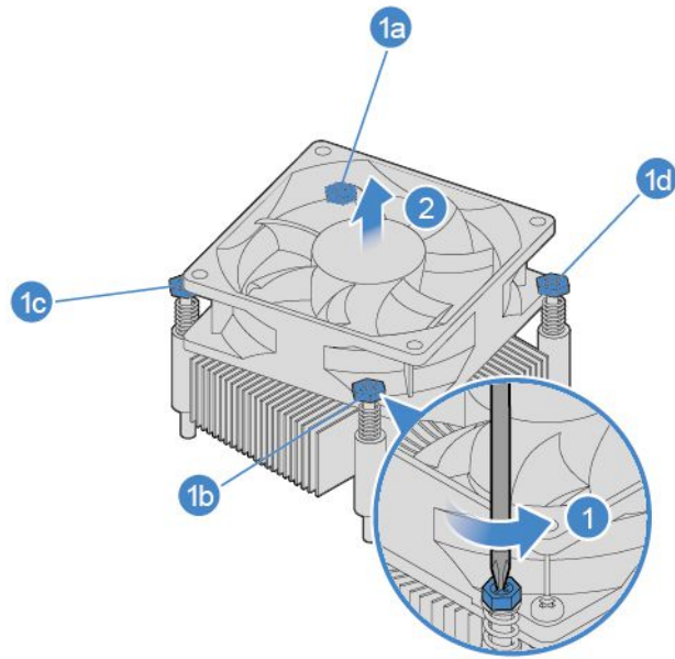
図 11. ヒートシンクおよびファンの取り外し
