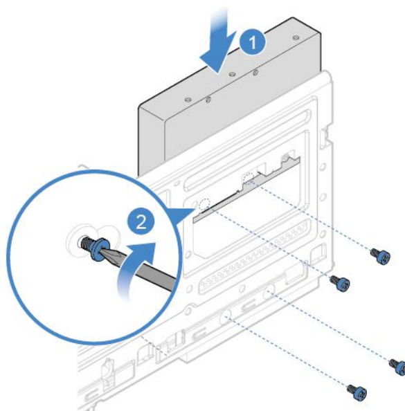
図 16. 3.5 型セカンダリー・ストレージ・ドライブの取り付け
