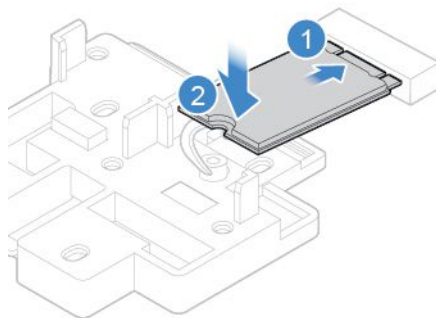
図47. M.2 ソリッド・ステート・ドライブの取り付け
