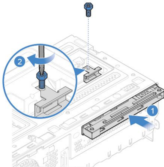
図8. 光学式ドライブ・ブラケットの取り付け
