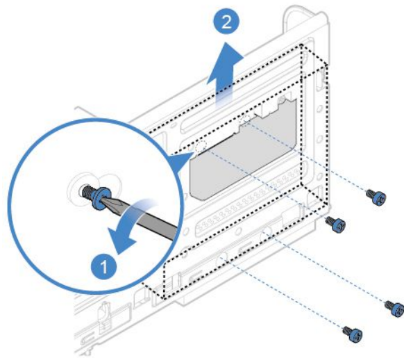
図 15. 3.5 型セカンダリー・ストレージ・ドライブの取り外し
