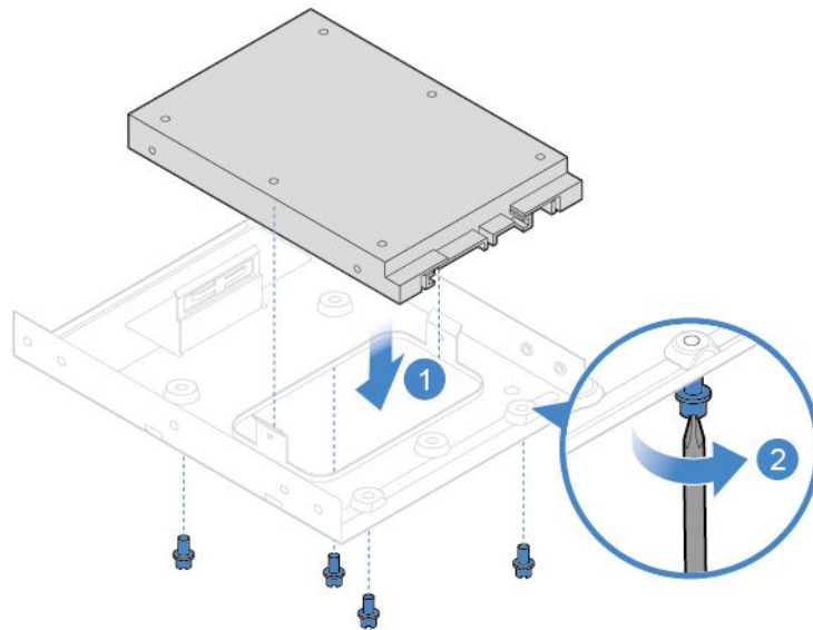
図 18. 2.5 型ストレージ・ドライブのストレージ・コンバーターへの取り付け
