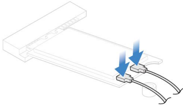
図 39. Wi-Fi アンテナ・ケーブルの接続
