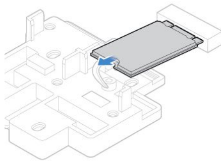
図46. M.2 ソリッド・ステート・ドライブの取り外し
