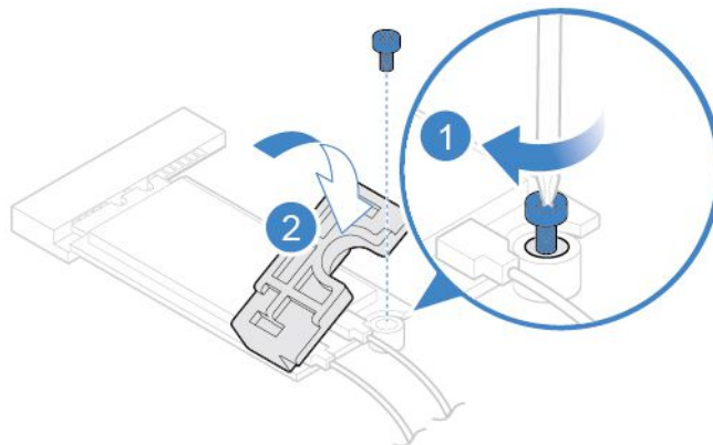
図 40. Wi-Fi カード・シールドの取り付け
