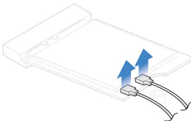
図30. Wi-Fi アンテナ・ケーブルの取り外し
