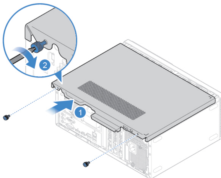
Figure 2. Remise en place du carter de l'ordinateur
