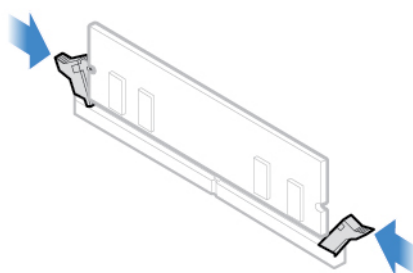
Figure 22. Fixation d'un module de mémoire avec les loquets
