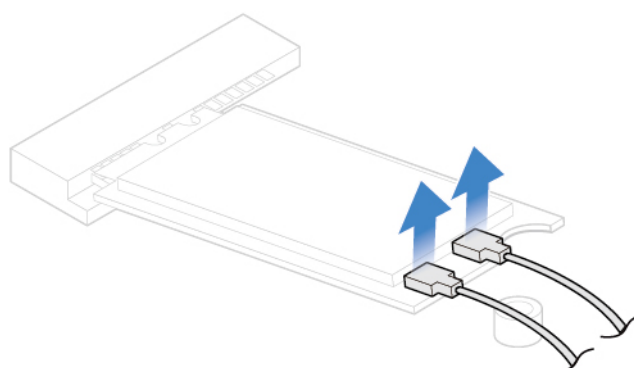
Figure 36. Débrancher les câbles d'antenne Wi-Fi
