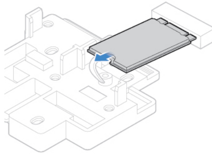
Abbildung 46. M.2-Solid-State-Laufwerk entfernen
