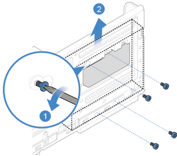
Abbildung 15. Sekundäres 3,5-Zoll-Speicherlaufwerk entfernen
