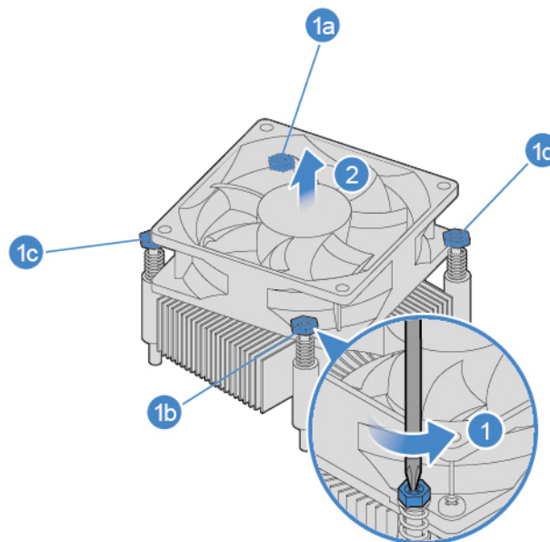
Abbildung 11. Kühlkörper- und Lüftungsbaugruppe entfernen
