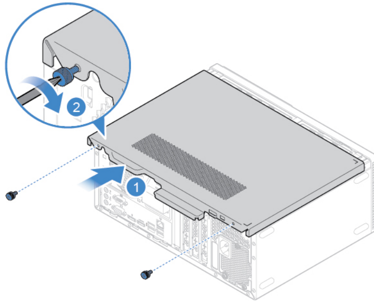
Abbildung 2. Computerabdeckung wieder anbringen
