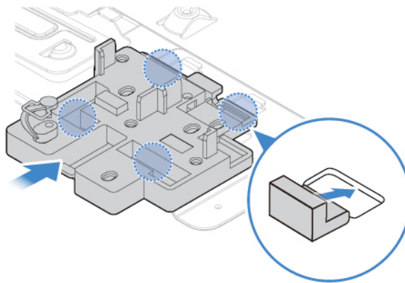
Abbildung 50. Halterung des M.2-Solid-State-Laufwerks installieren
