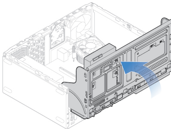
Abbildung 10. Laufwerkpositionsbaugruppe nach unten klappen
