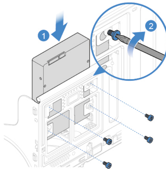
Abbildung 14. Primäres 3,5-Zoll-Speicherlaufwerk installieren
