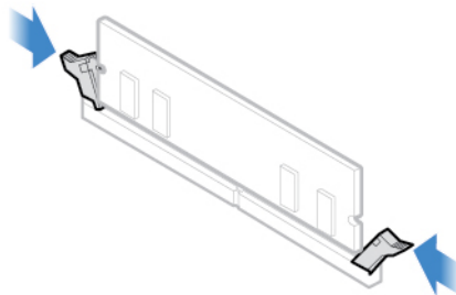
Abbildung 22. Speichermodul mit den Verriegelungen befestigen
