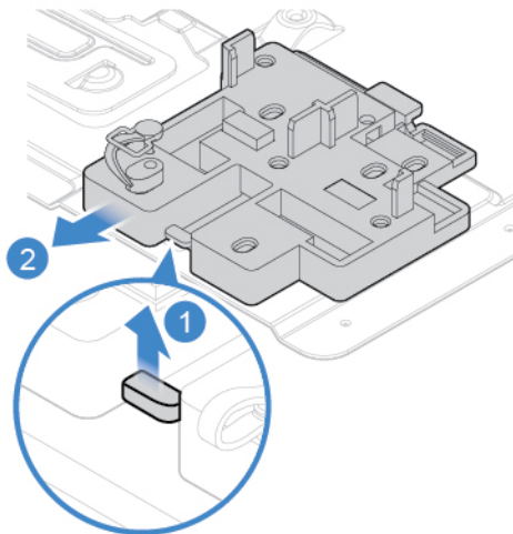
Abbildung 49. Halterung des M.2-Solid-State-Laufwerks entfernen
