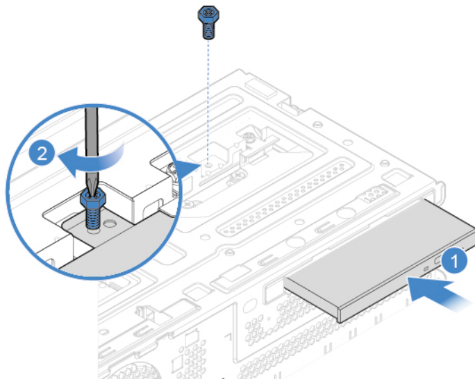
Abbildung 6. Optisches Laufwerk installieren
