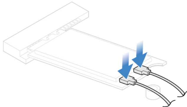
Abbildung 39. Wi-Fi-Antennenkabel anschließen
