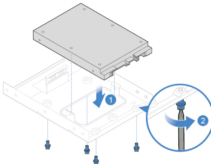
Abbildung 18. 2,5-Zoll-Speicherlaufwerk in den Speicherkonverter einbauen
