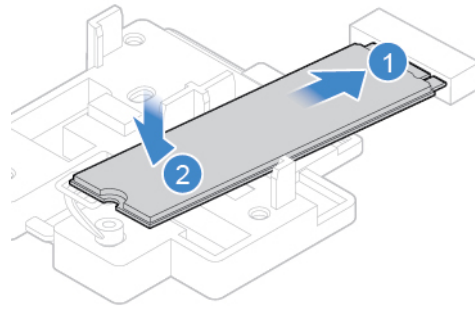
Abbildung 43. M.2-Solid-State-Laufwerk installieren
