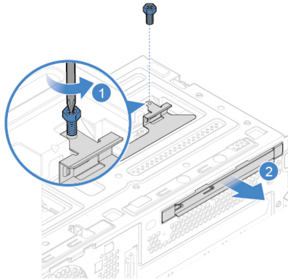
Abbildung 7. Halterung für optisches Laufwerk entfernen
