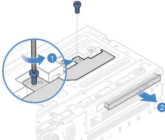
Abbildung 5. Optisches Laufwerk entfernen
