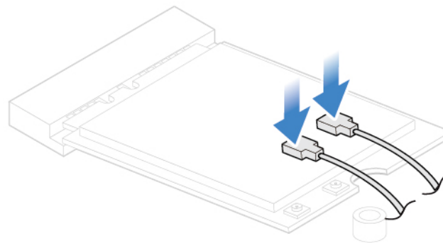
Abbildung 33. Wi-Fi-Antennenkabel anschließen
