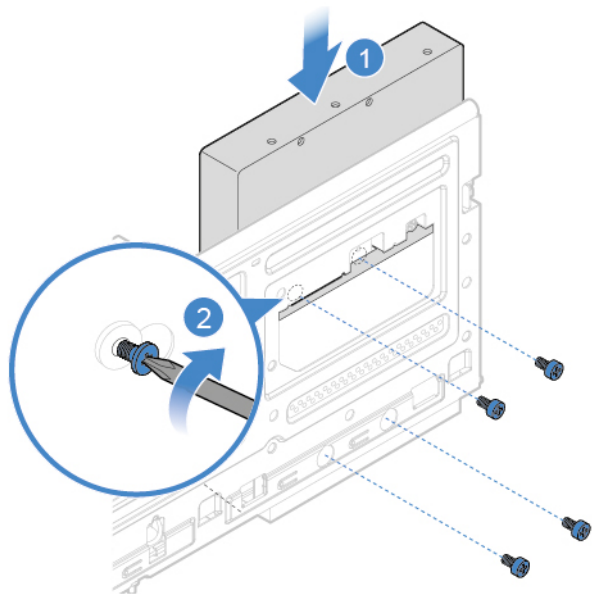
Abbildung 16. Sekundäres 3,5-Zoll-Speicherlaufwerk installieren
