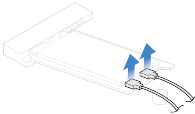
Abbildung 36. Wi-Fi-Antennenkabel entfernen
