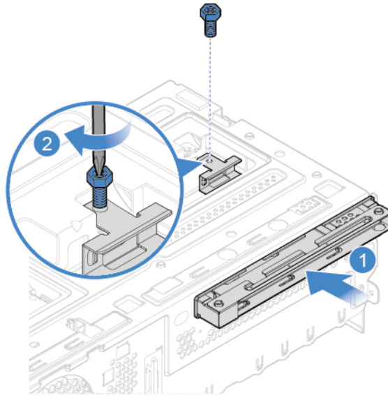
Abbildung 8. Halteklammer des optischen Laufwerks installieren
