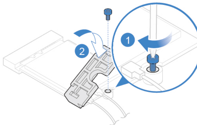
Abbildung 34. Abdeckung der Wi-Fi-Karte installieren
