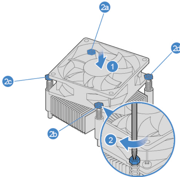
Abbildung 12. Kühlkörper- und Lüftungsbaugruppe installieren
