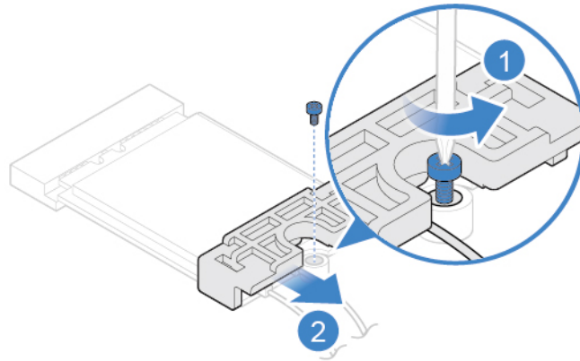
Abbildung 29. Abdeckung der Wi-Fi-Karte entfernen
