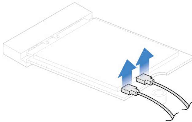
Abbildung 30. Wi-Fi-Antennenkabel entfernen
