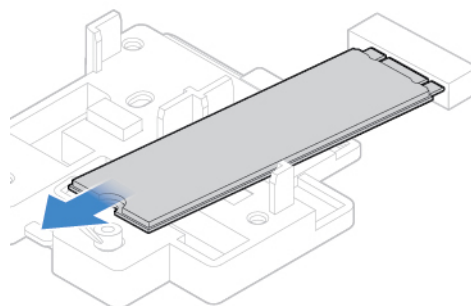
Abbildung 42. M.2-Solid-State-Laufwerk entfernen
