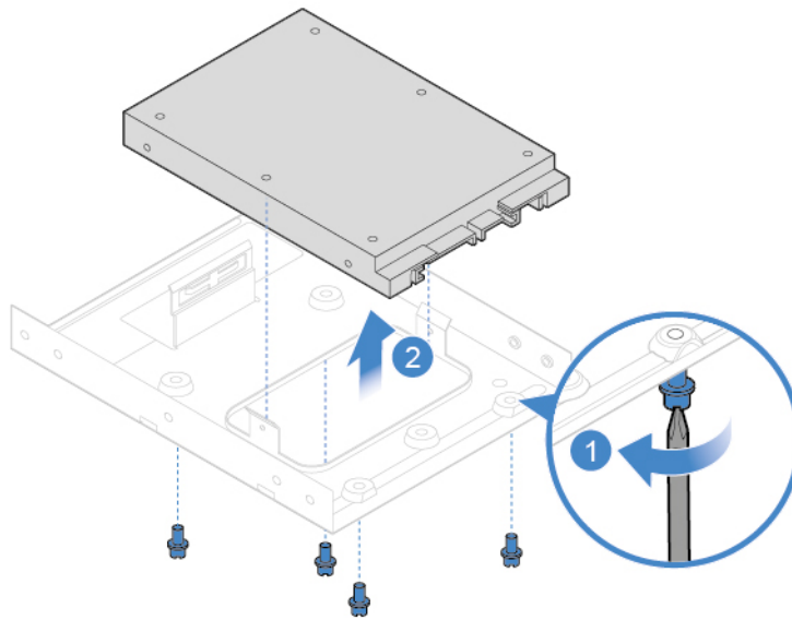
Abbildung 17. Das 2,5-Zoll-Speicherlaufwerk aus dem Speicherkonverter entfernen
