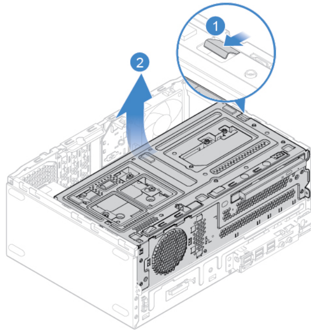
Abbildung 9. Laufwerkpositionsbaugruppe nach oben klappen
