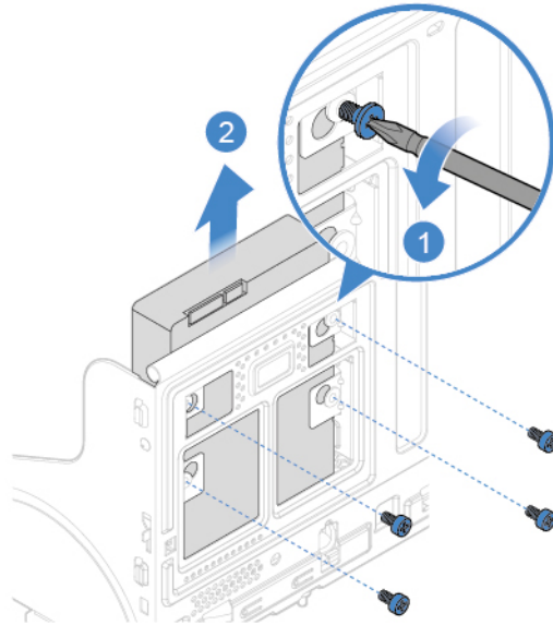
Abbildung 13. Primäres 3,5-Zoll-Speicherlaufwerk entfernen
