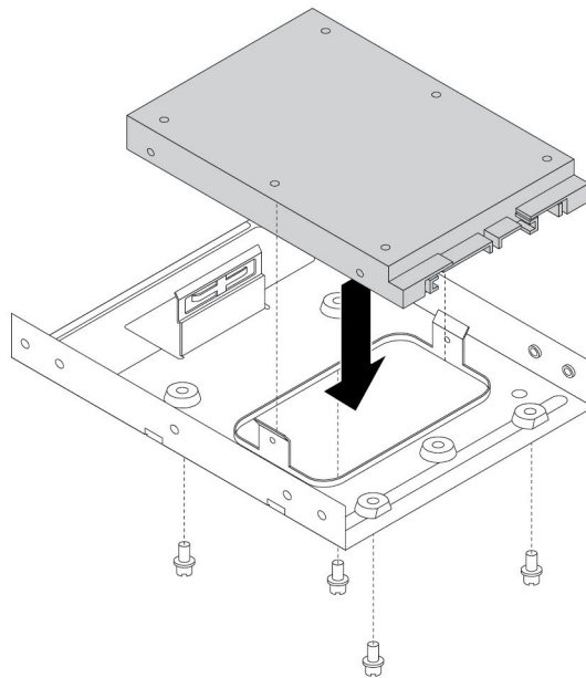
그림 74. 저장 컨버터에 새 솔리드 스테이트 드라이브 장착
