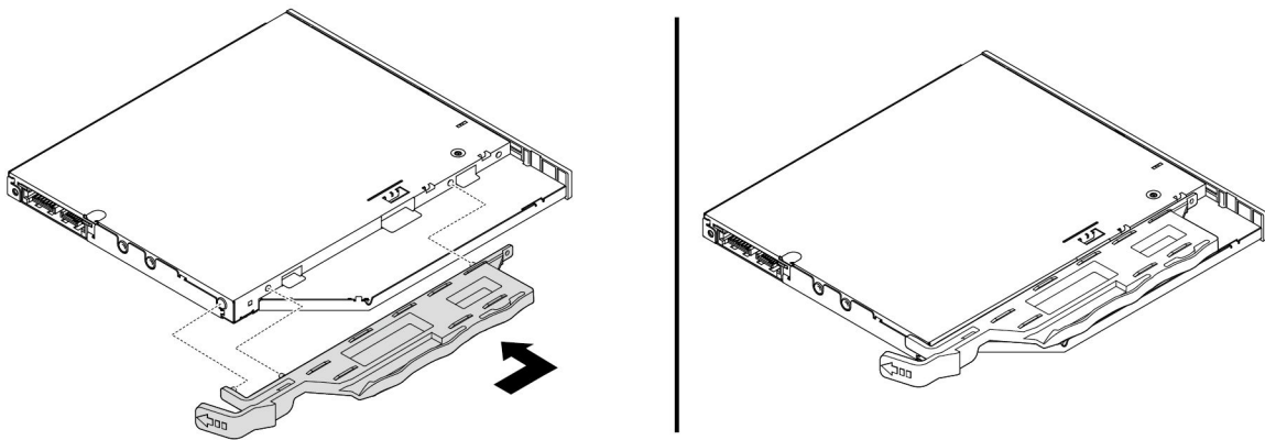
그림 48. 새 슬림 광 드라이브에 브래킷 설치
