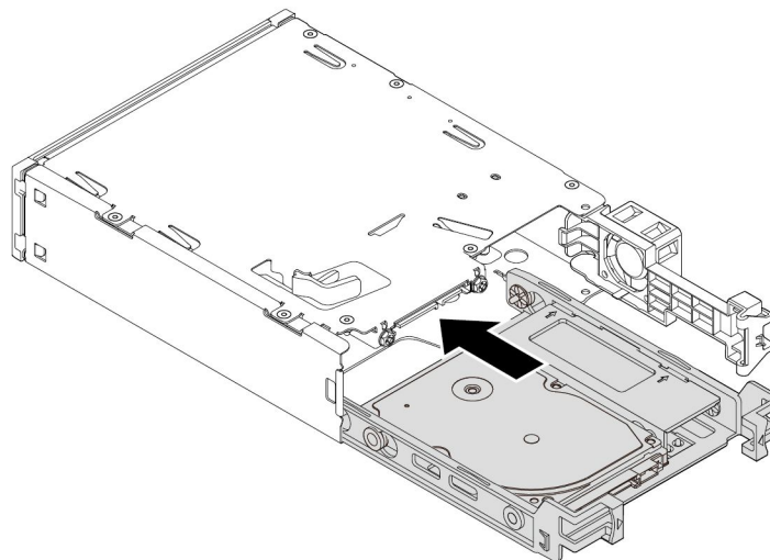
그림 60. 새 2.5인치 내부 저장 장치 드라이브를 키트 안에 밀어넣기
