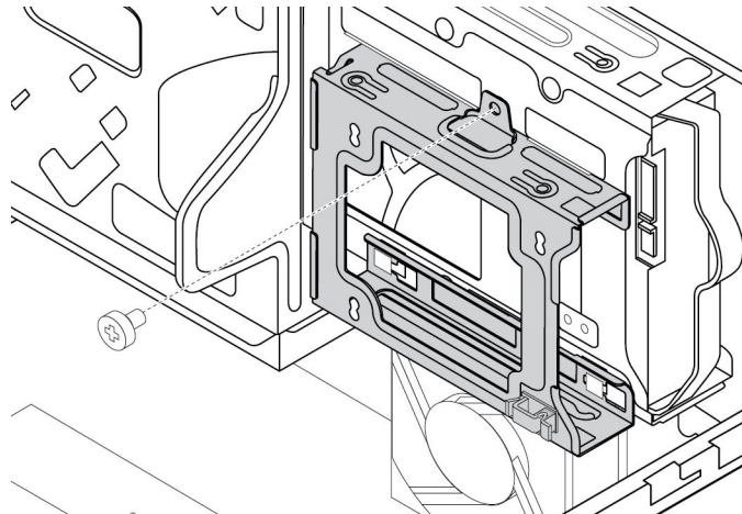
그림 93. 나사를 조여 보조 하드 디스크 드라이브 케이지 고정
