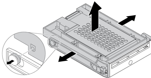
그림 38. 브래킷에서 2.5인치 저장 장치 드라이브 제거
