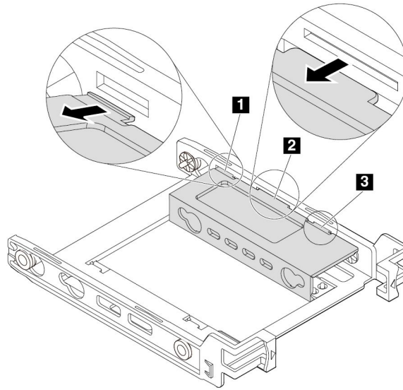
그림 67. 탭 1, 2 및 3을 해당 슬롯에서 해제
