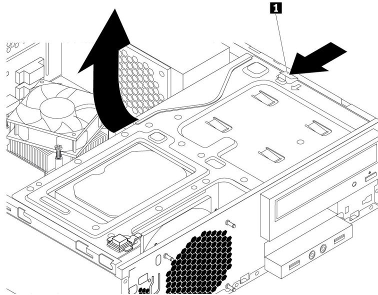
그림 85. 드라이브 베이 어셈블리 위로 당기기
