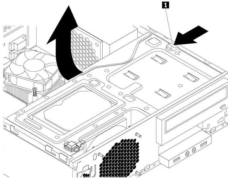
그림 89. 드라이브 베이 어셈블리 위로 당기기
