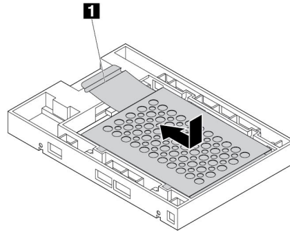
그림 43. 컨버터의 플라스틱 프레임에 금속 브래킷 설치
