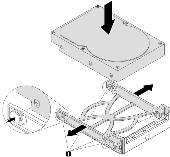
그림 34. 브래킷에 3.5인치 저장 장치 드라이브 설치
