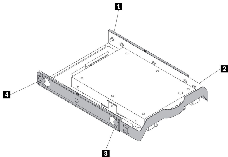
그림 71. 저장 장치 드라이브 브래킷에 솔리드 스테이트 드라이브가 있는 저장 장치 컨버터 설치
