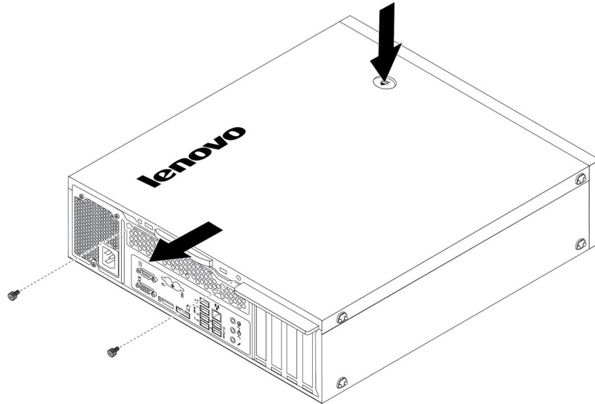
그림 10. 컴퓨터 덮개 제거
