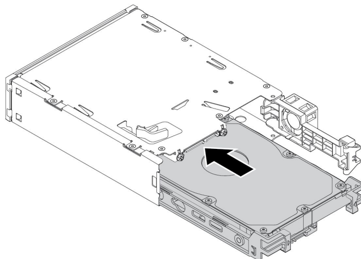
그림 54. 새 3.5인치 내부 저장 장치 드라이브를 키트 안에 밀어넣기
