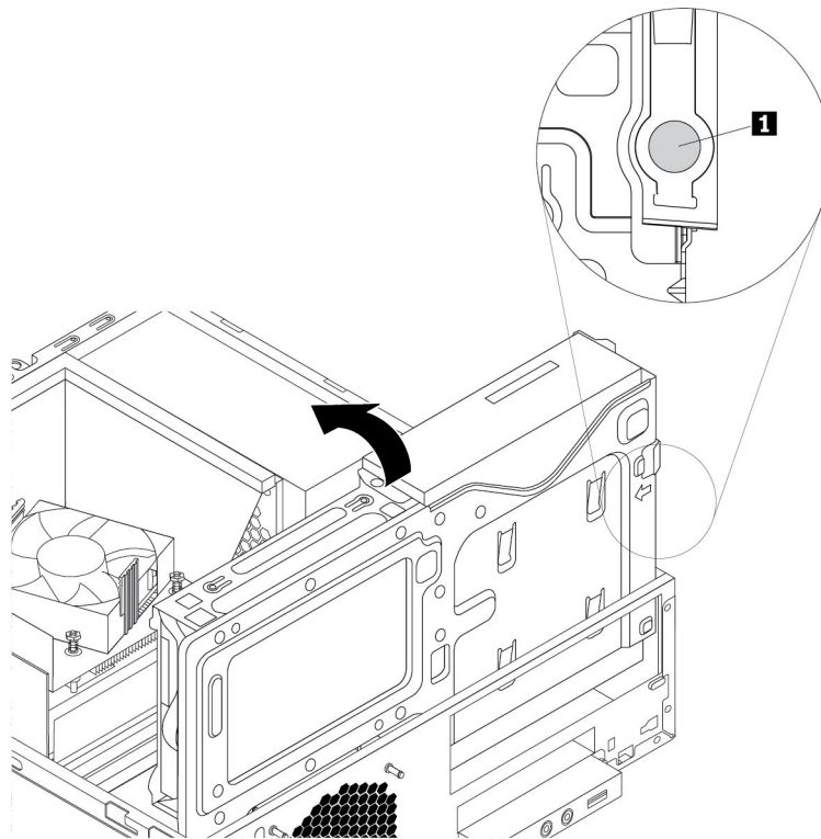
그림 96. 드라이브 베이 어셈블리 아래로 당기기
