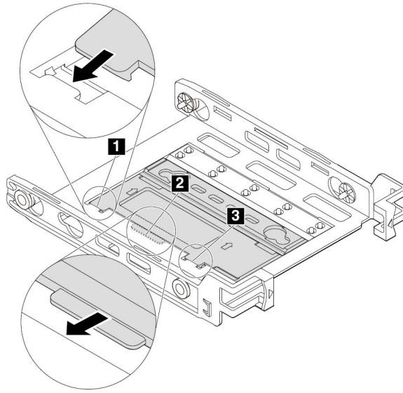
그림 69. 탭 1 및 3을 해당 슬롯에 삽입하기
