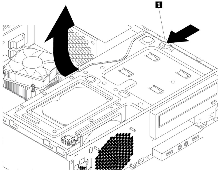
그림 80. 드라이브 베이 어셈블리 위로 당기기
