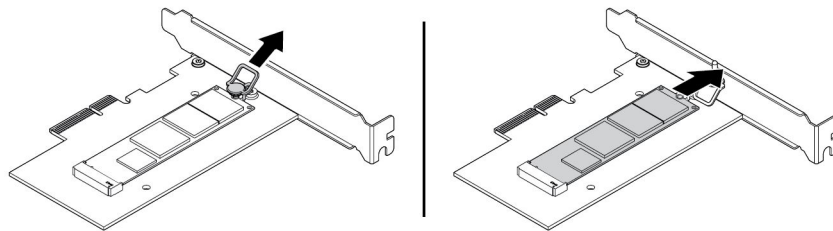
그림 17. M.2 솔리드 스테이트 드라이브 제거
