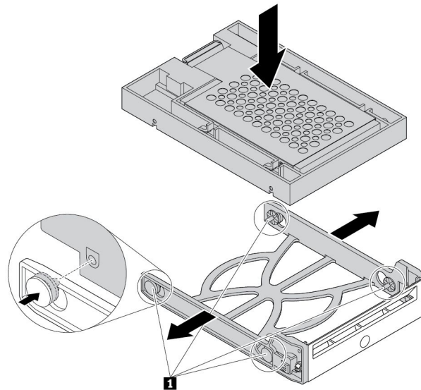
그림 44. 플라스틱 브래킷에 2.5인치 저장 장치 드라이브와 조립된 컨버터 장착
