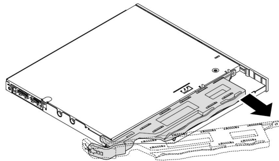
그림 47. 슬림 광 드라이브에서 브래킷 제거
