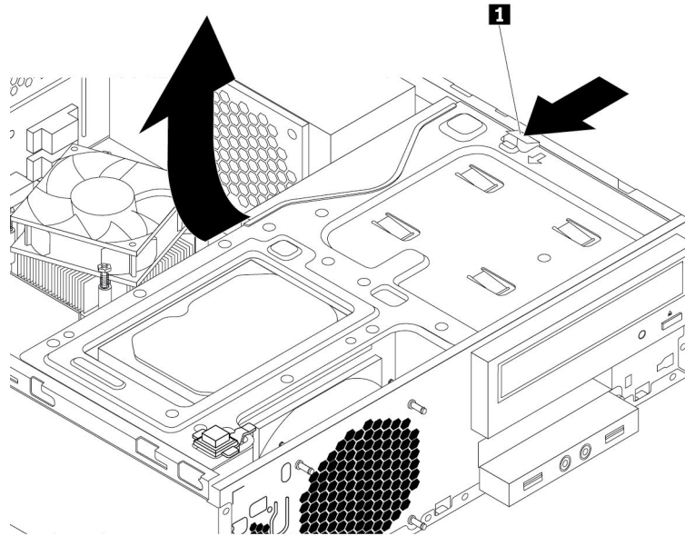
그림 27. 드라이브 베이 어셈블리 위로 당기기
