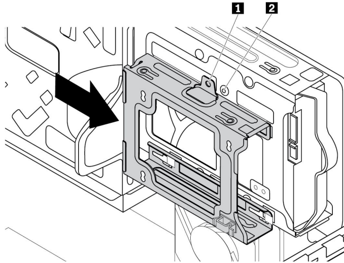
그림 92. 보조 하드 디스크 드라이브 케이지 설치
