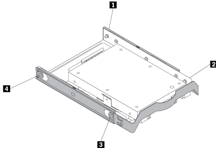
그림 75. 새 솔리드 스테이트 드라이브를 갖춘 저장 컨버터를 저장 드라이브 브래킷에 장착
