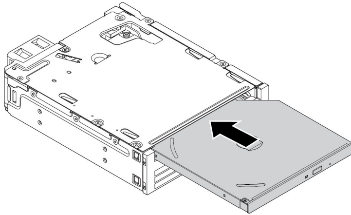
그림 49. 키트에 슬림 광 드라이브 설치
