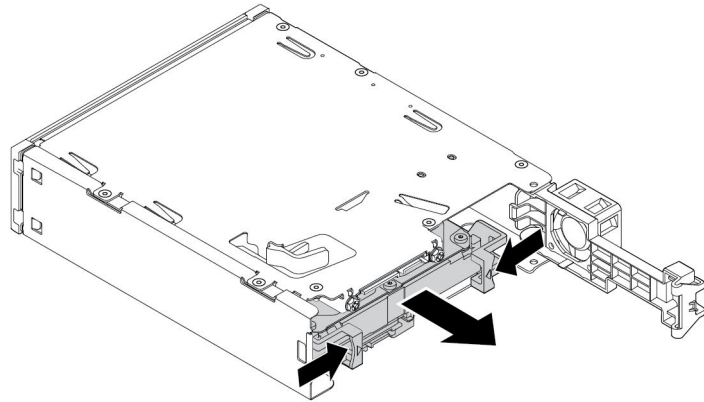
그림 51. 뒷면에서 3.5인치 내부 저장 장치 드라이브 제거
