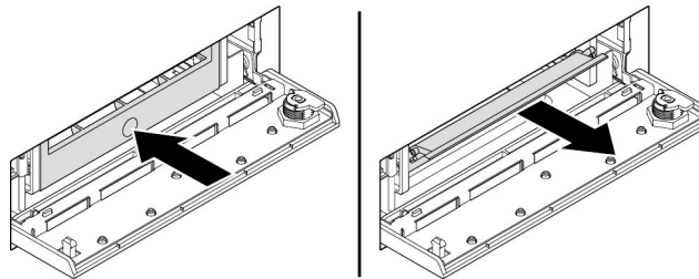
그림 32. 앞면 액세스 저장 장치 엔클로저에서 브래킷 제거
