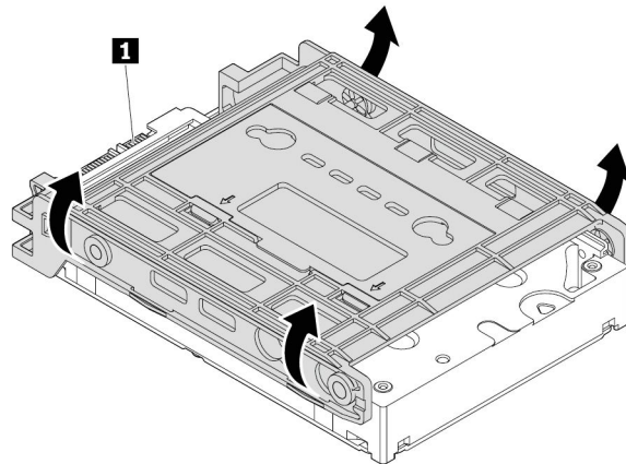
그림 52. 브래킷의 두 측면을 구부려 3.5인치 내부 저장 장치 드라이브를 제거하십시오
