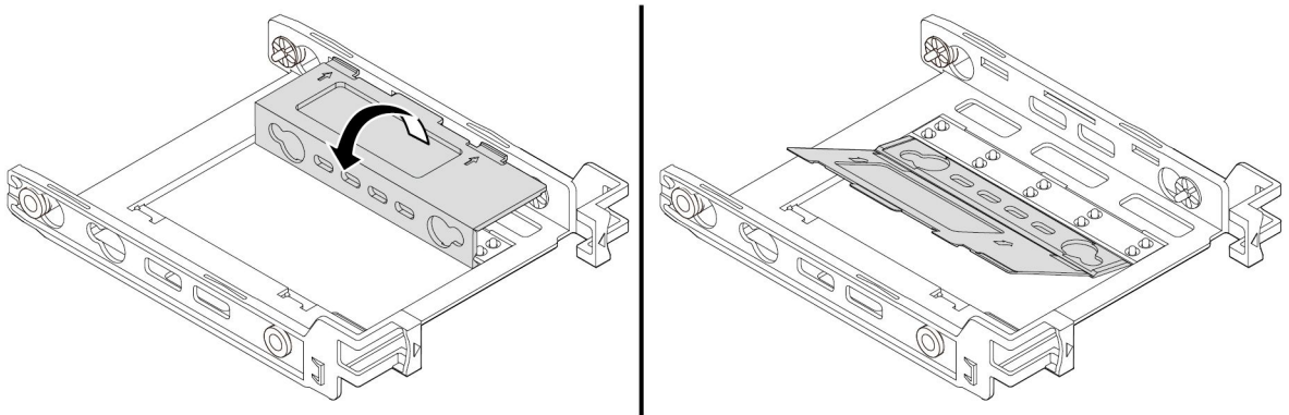
그림 68. 브래킷 펴기
