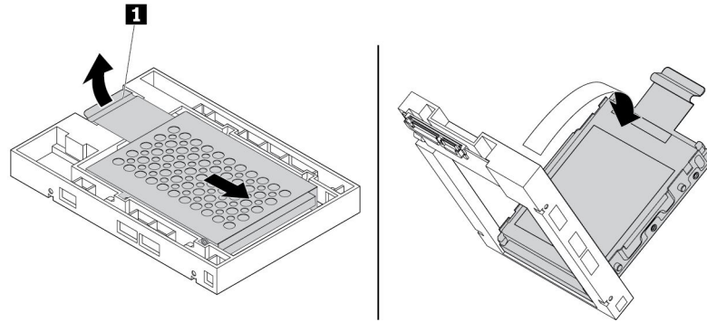
그림 39. 컨버터의 플라스틱 프레임에서 금속 브래킷 제거
