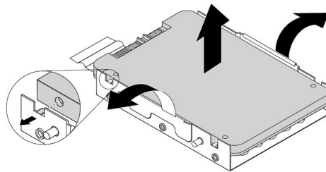
그림 40. 금속 브래킷에서 저장 장치 드라이브 제거
