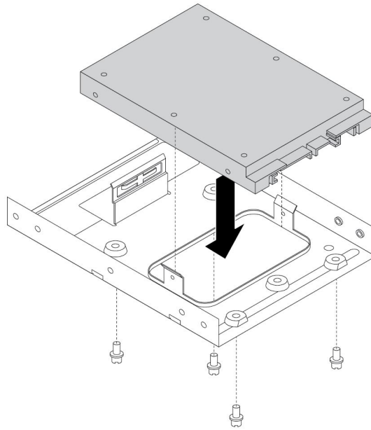
그림 70. 저장 컨버터에 솔리드 스테이트 드라이브 장착
