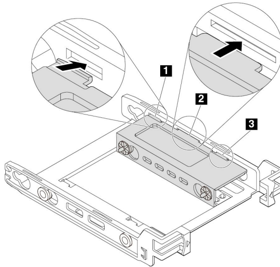
그림 65. 탭 1 및 3 을 해당 슬롯에 삽입하기
