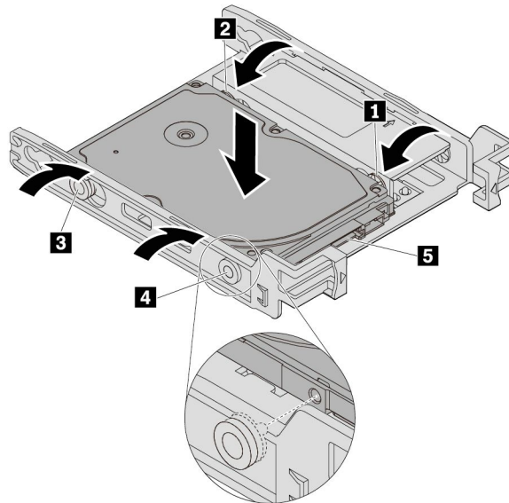
그림 59. 새로운 2.5인치 내부 저장 드라이브를 브래킷에 설치
