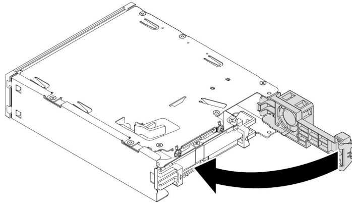
그림 61. 뒷면 덮개를 안쪽으로 돌리기
