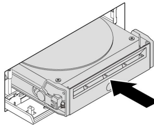
그림 35. 앞면 액세스 저장 장치 엔클로저에 3.5인치 저장 장치 드라이브 장착
