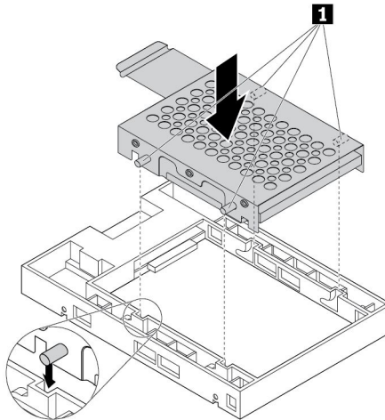
그림 42. 컨버터의 플라스틱 프레임에 금속 브래킷 삽입
