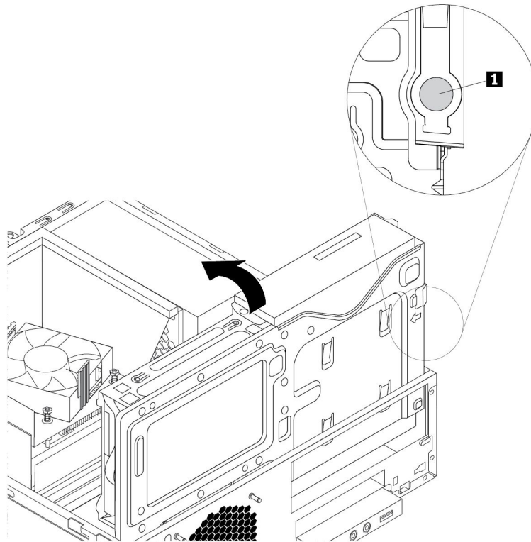
그림 83. 드라이브 베이 어셈블리 아래로 당기기
