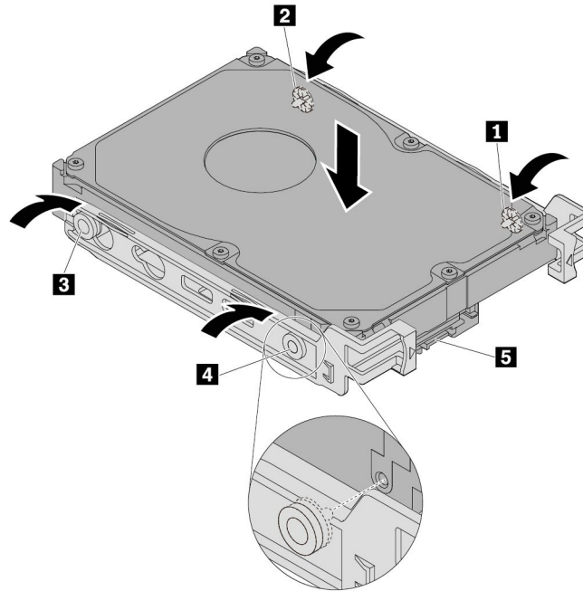
그림 53. 새로운 3.5인치 내부 저장 드라이브를 브래킷에 설치
