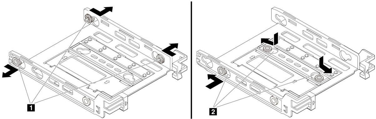
그림 62. 3개의 핀 제거 및 새 슬롯에 설치
