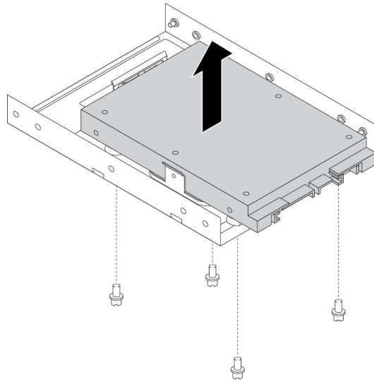
그림 73. 저장 장치 컨버터에서 솔리드 스테이트 드라이브 제거
