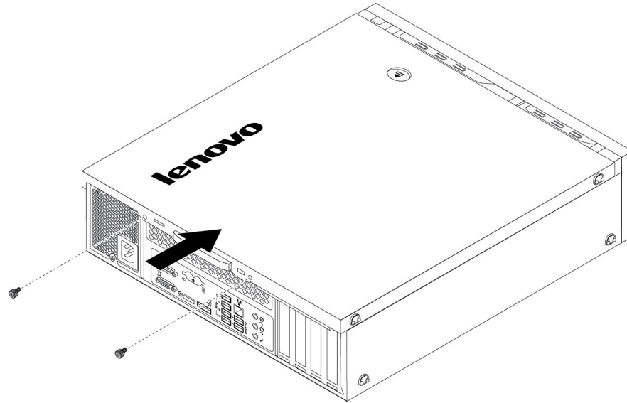
그림 97. 컴퓨터 덮개 다시 장착
