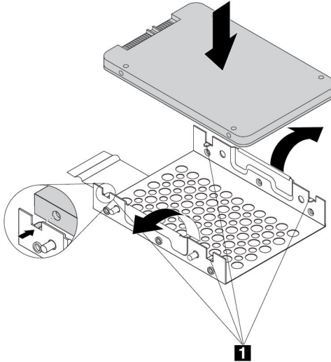
그림 41. 금속 브래킷에 2.5인치 저장 장치 드라이브 장착
