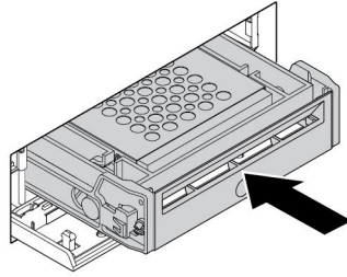
그림 45. 앞면 액세스 저장 장치 엔클로저에 2.5인치 저장 장치 드라이브와 조립된 브래킷 설치
