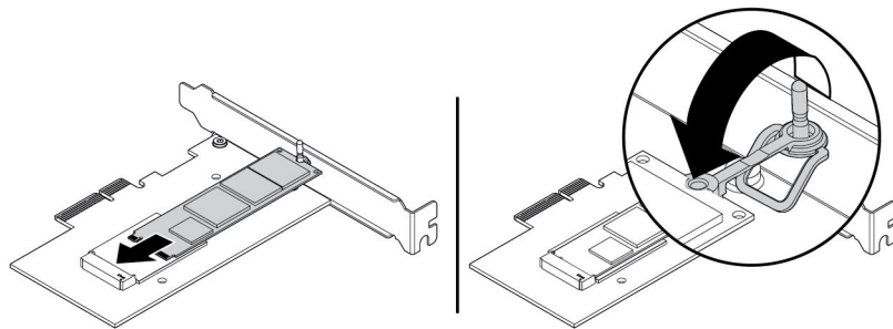
그림 19. M.2 솔리드 스테이트 드라이브 설치
