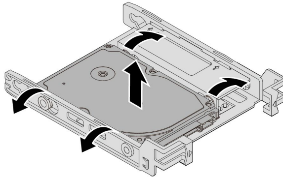
그림 58. 브래킷의 두 측면을 구부려 2.5인치 내부 저장 장치 드라이브를 제거하십시오
