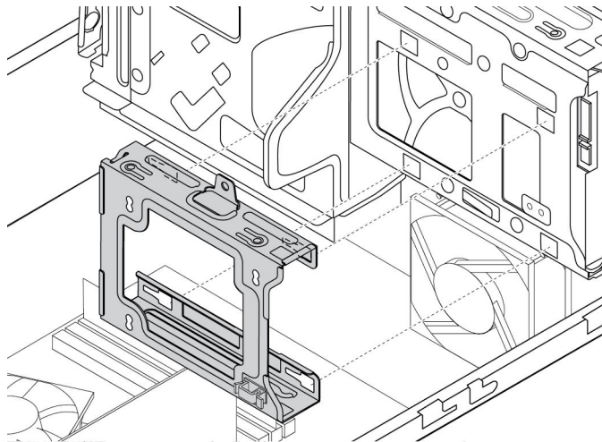
그림 91. 기본 하드 디스크 드라이브 베이의 밑면에 케이스 놓기
