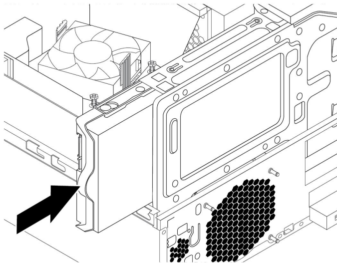
그림 88. 기본 하드 디스크 드라이브 설치
