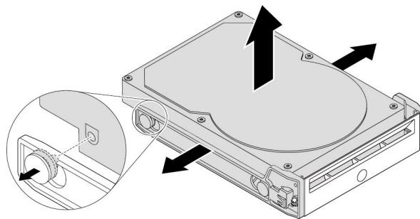
그림 33. 브래킷에서 3.5인치 저장 장치 드라이브 제거
