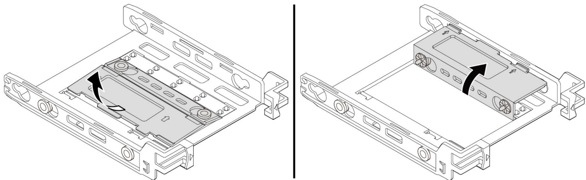
그림 64. 브래킷 접기
