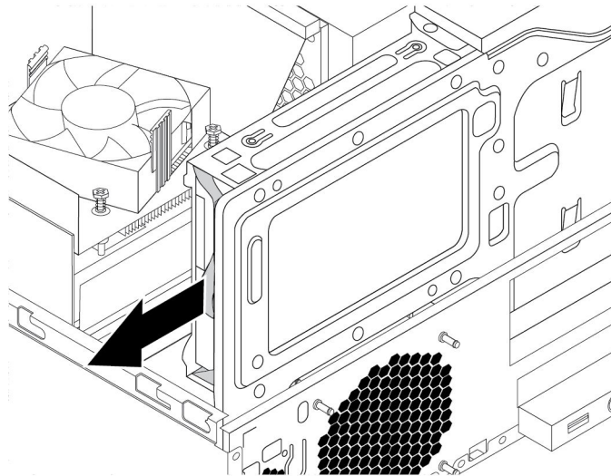
그림 86. 기본 하드 디스크 드라이브 제거
