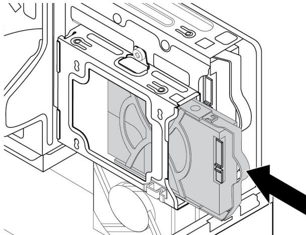
그림 95. 보조 하드 디스크 드라이브 설치
