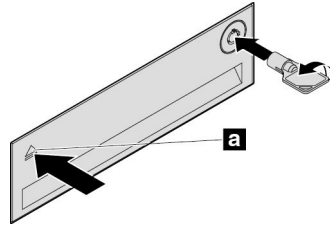
그림 36. 앞면 액세스 저장 엔클로저의 덮개 열기
