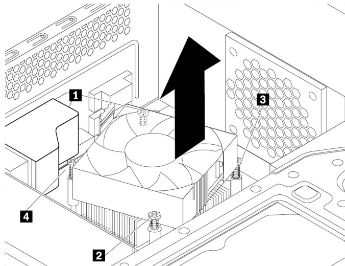
그림 77. 방열판 및 팬 어셈블리를 고정하는 나사
