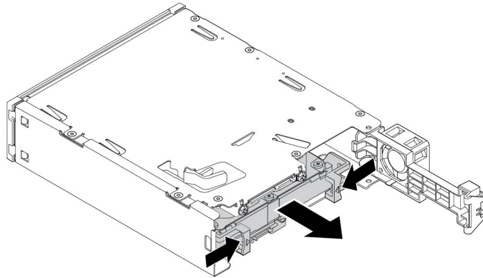
그림 57. 뒷면에서 2.5인치 내부 저장 장치 드라이브 제거
