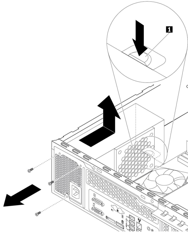
그림 81. 전원 공급 장치 어셈블리 제거
