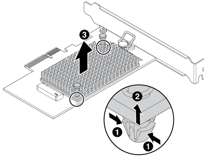
그림 16. M.2 솔리드 스테이트 드라이브 어댑터에서 방열판을 제거
