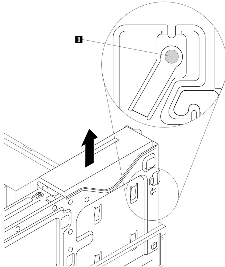
그림 28. 광 드라이브 제거
