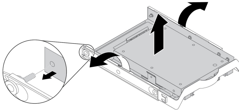
그림 72. 3.5인치 저장 드라이브 브래킷에서 저장 컨버터 제거
