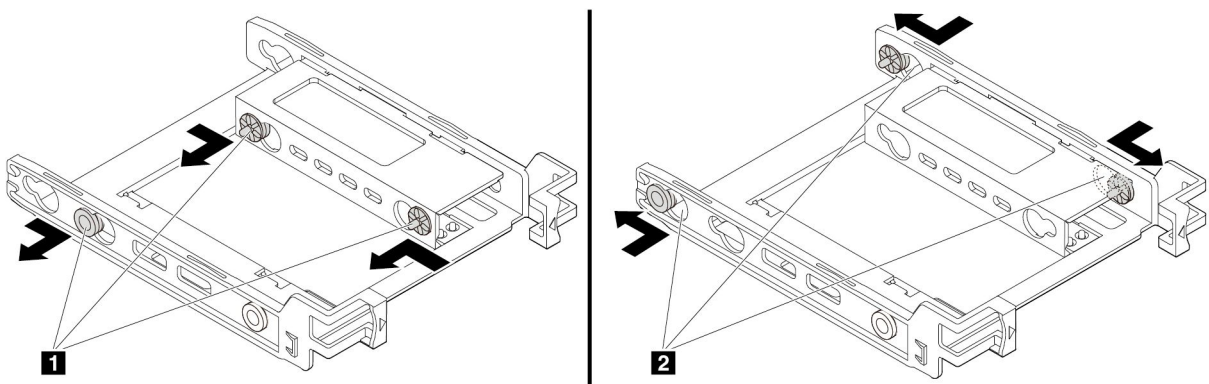
그림 66. 3개의 핀 제거 1 및 새 슬롯에 설치 2
