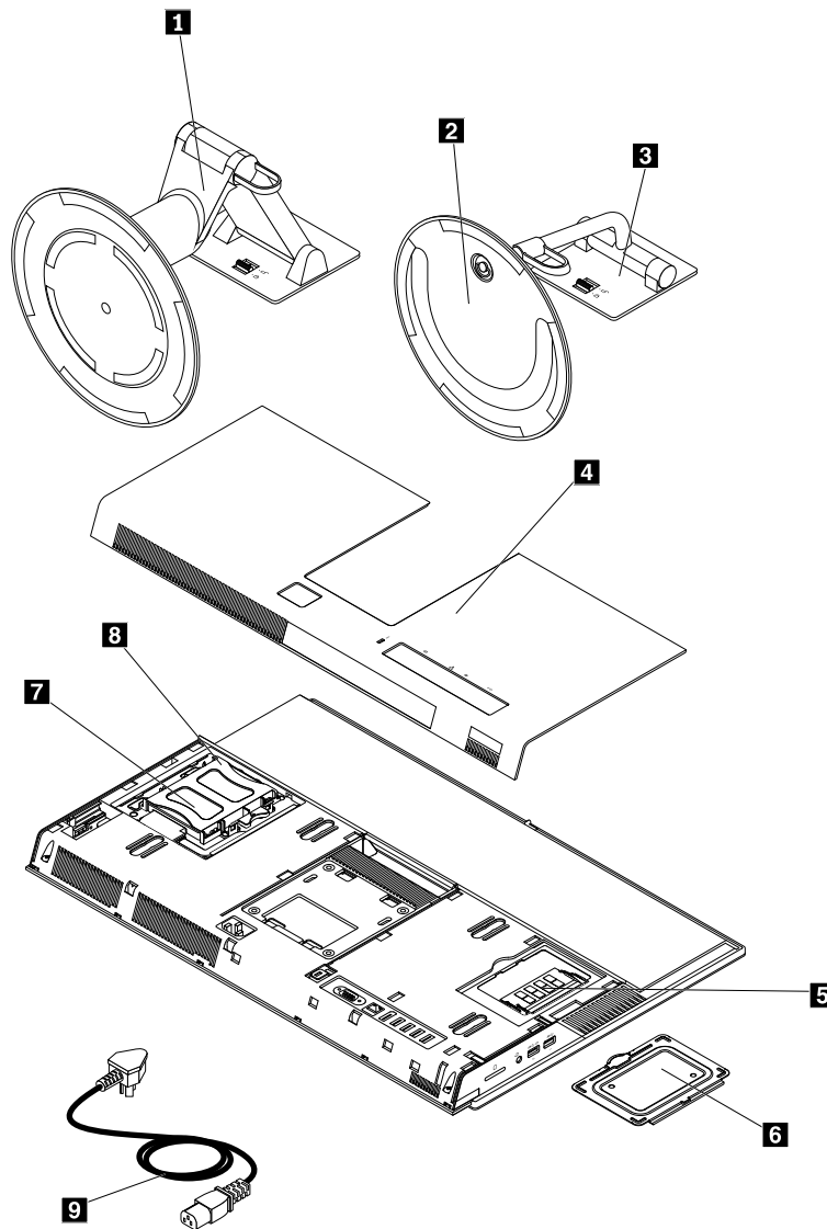
Abbildung 3. Computerkomponenten
