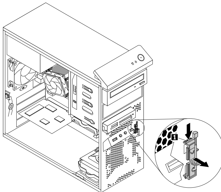
Рис. 71. Снятие датчика температуры
