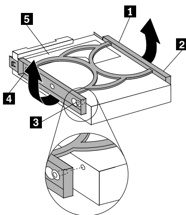
Рис. 58. Установка жесткого диска в крепежную скобку
