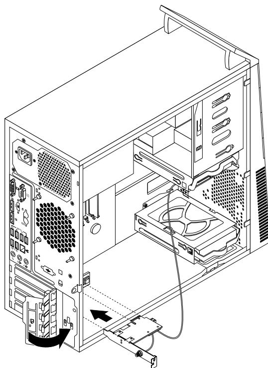
Рис. 84. Установка карты контроллера Wi-Fi
