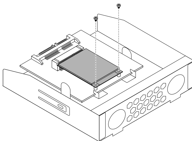
Рис. 49. Снятие винтов, крепящих твердотельный диск mSATA
