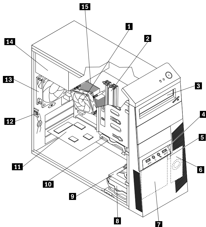
Рис. 4. Расположение компонентов
