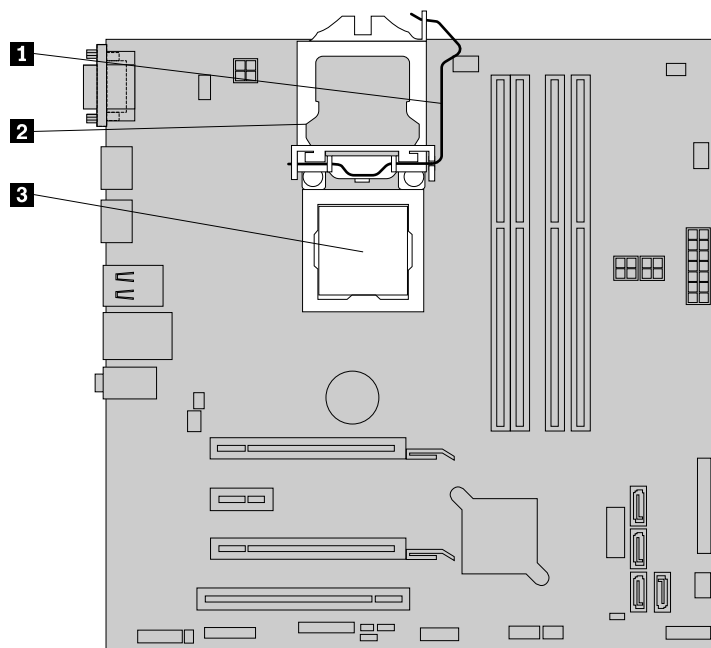
Рис. 42. Доступ к микропроцессору
