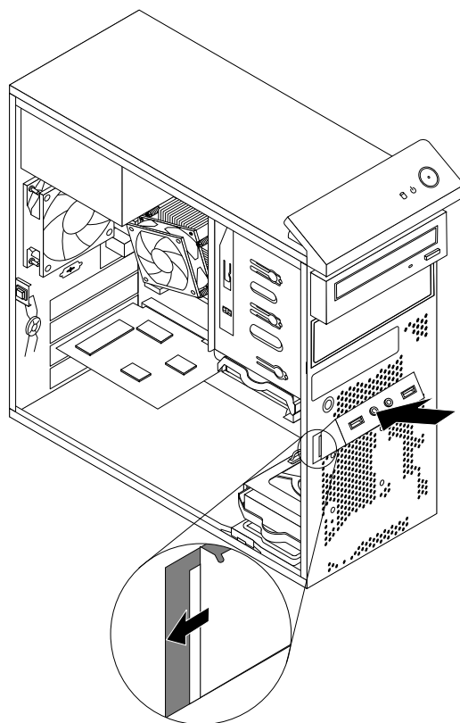
Рис. 67. Установка переднего блока аудиоразъема и USB-портов
