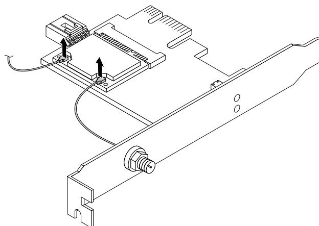
Рис. 78. Отключение кабелей антенн Wi-Fi
