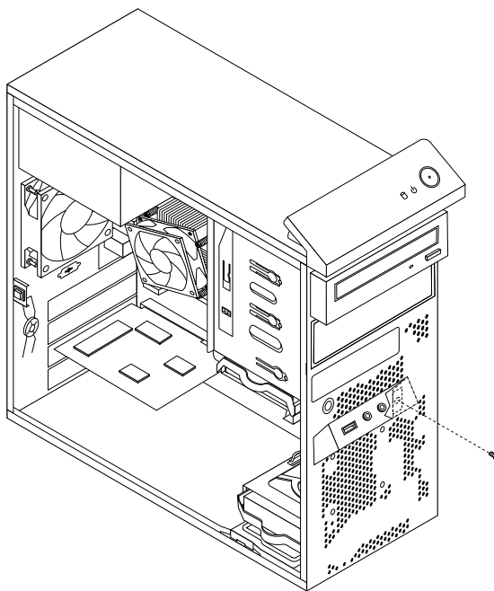
Рис. 68. Установка винта для закрепления переднего блока аудиоразъемов и разъемов USB
