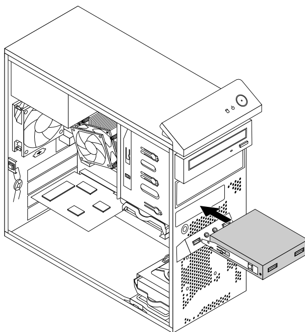
Рис. 37. Установка переднего блока разъемов USB
