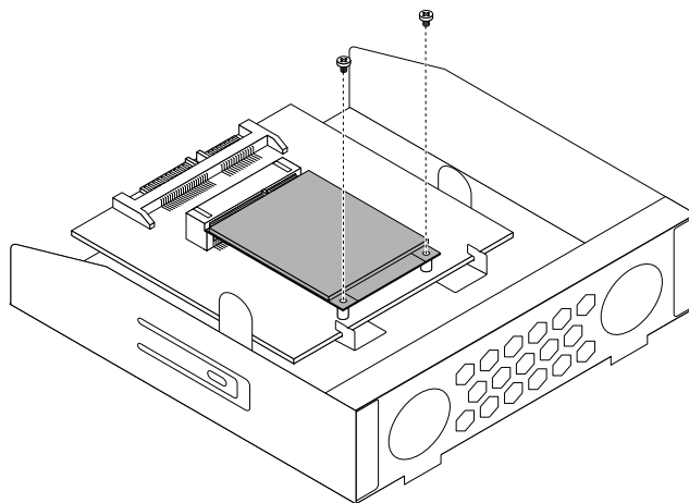
Рис. 52. Затягивание винтов, крепящих твердотельный диск mSATA
