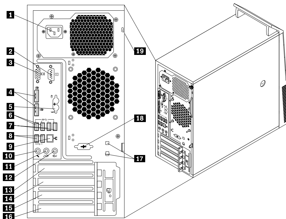
Рис. 2. Расположение разъемов на задней панели компьютера ThinkCentre M93/p
