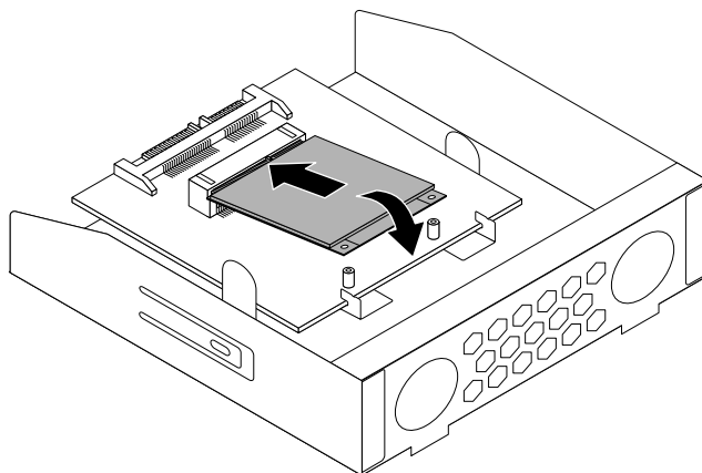
Рис. 51. Установка твердотельного диска mSATA в адаптер
