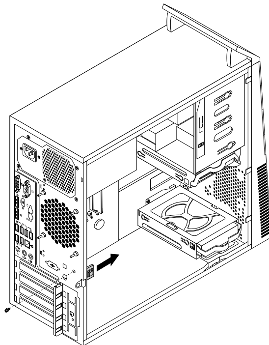
Рис. 73. Отсоединение датчика установленного кожуха
