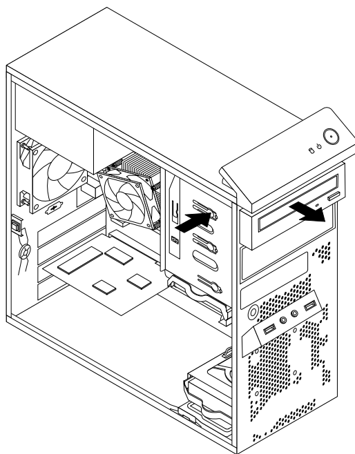
Рис. 20. Снятие дисковода для оптических дисков
