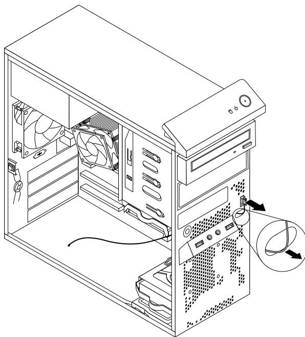
Рис. 89. Снятие передней антенны Wi-Fi
