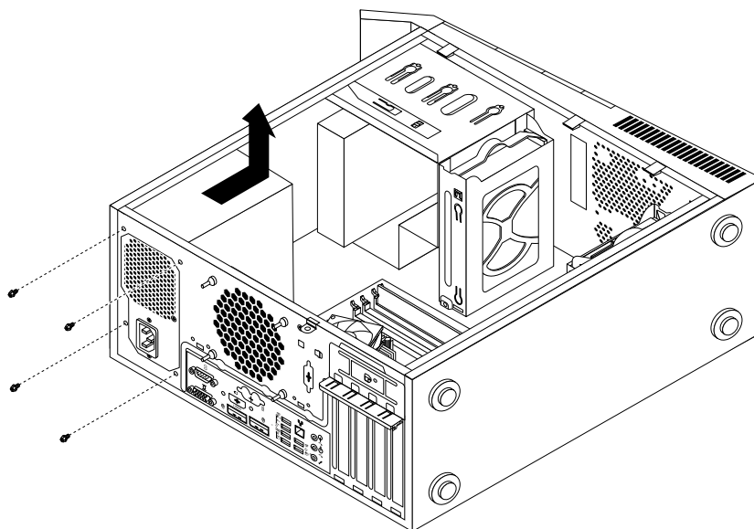
Рис. 40. Отверните винты, закрепляющие блок питания
