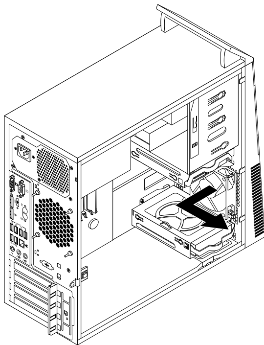
Рис. 62. Снятие переднего блока вентилятора
