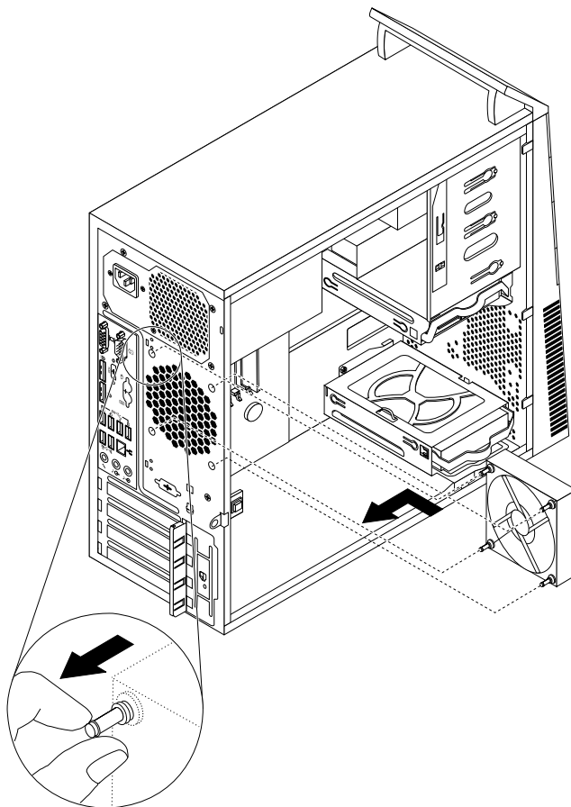
Рис. 65. Установка заднего блока вентилятора.
