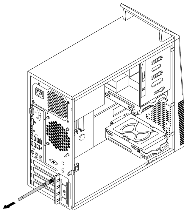
Рис. 86. Снятие задней антенны Wi-Fi
