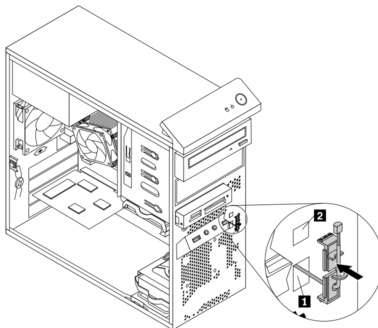
Рис. 72. Установка нового датчика температуры
