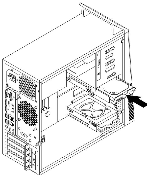
Рис. 56. Установка основного жесткого диска
