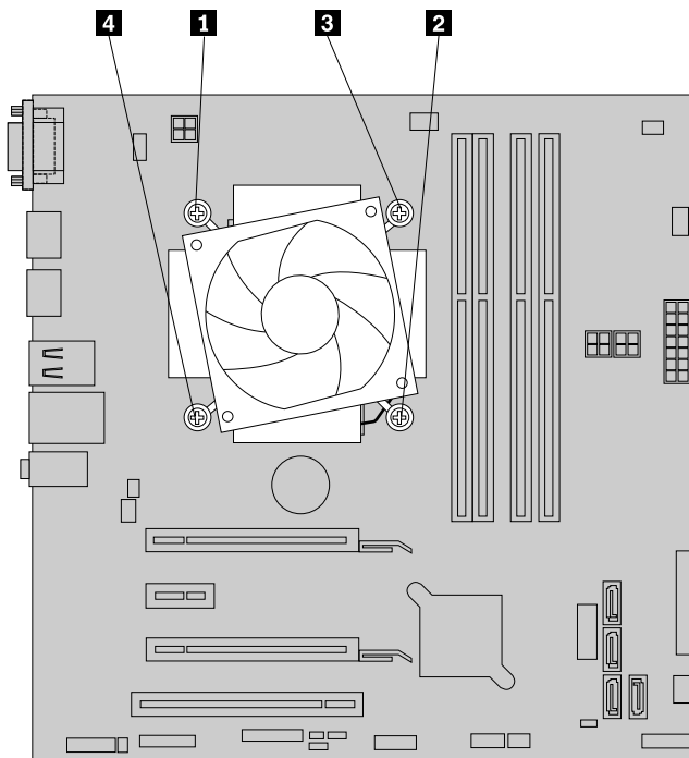
Рис. 41. Снятие блока радиатора и вентилятора
