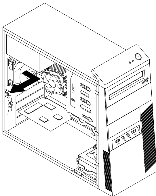
Рис. 64. Снятие заднего блока вентилятора
