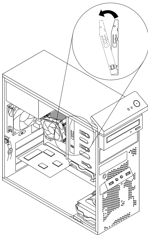
Рис. 24. Снятие крепежной скобы считывателя карт
