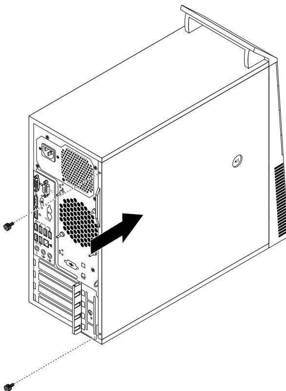
Рис. 91. Как поставить на место кожух компьютера
