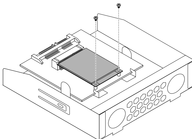
Рис. 46. Затягивание винтов, крепящих твердотельный диск mSATA
