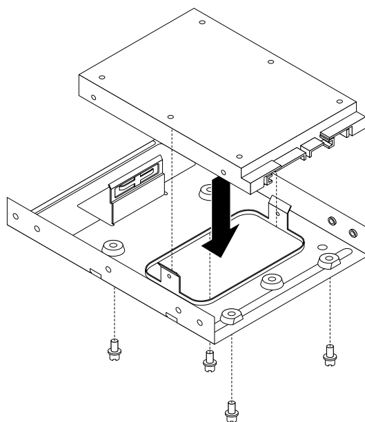
Рис. 60. Установка твердотельного диска в адаптер
