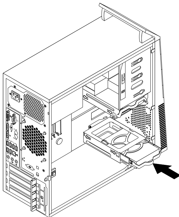
Рис. 59. Установка дополнительного жесткого диска
