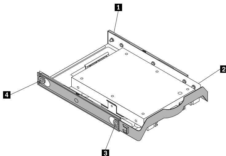
Рис. 61. Установка твердотельного диска с адаптером в крепежную скобу для жесткого диска
