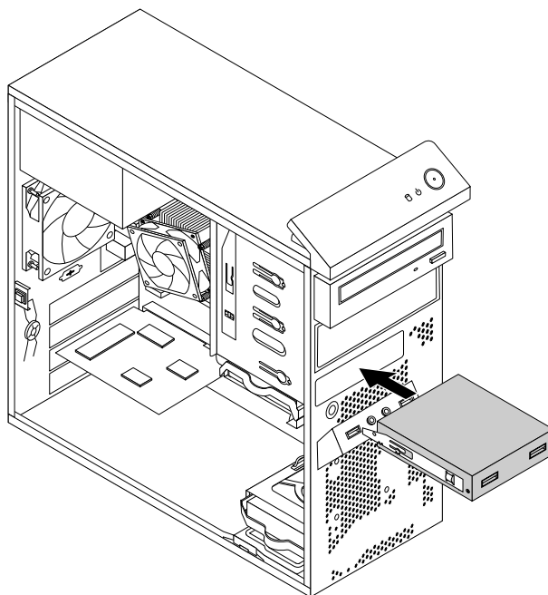
Рис. 33. Установка переднего блока разъемов USB
