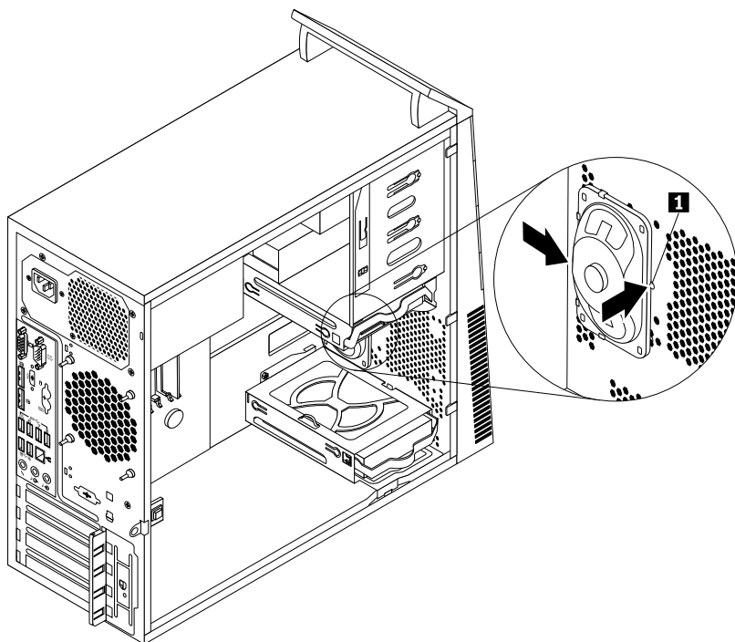
Рис. 69. Как снять внутренний динамик
