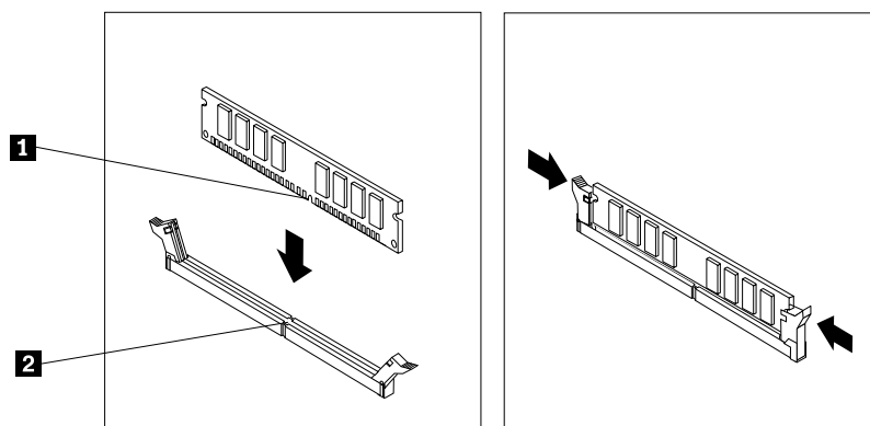
Рис. 19. Установка модуля памяти
