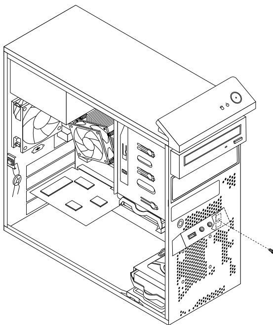
Рис. 66. Снятие переднего блока аудиоразъемов и USB
