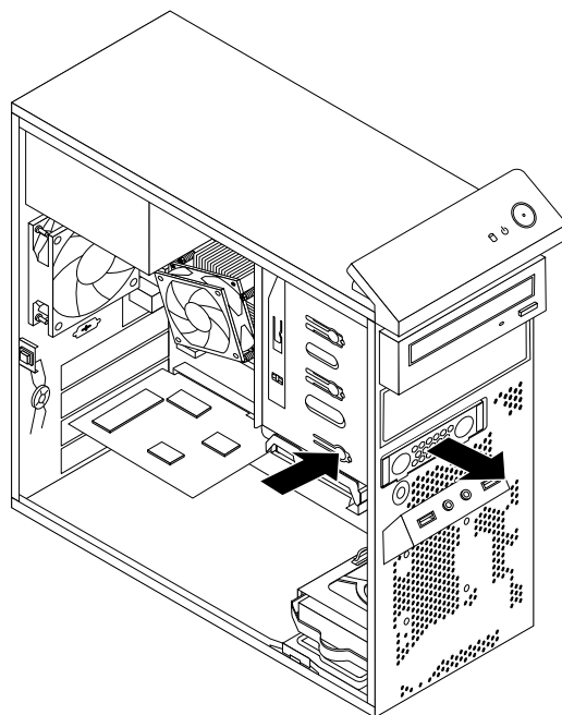
Рис. 48. Извлечение адаптера твердотельного диска mSATA
