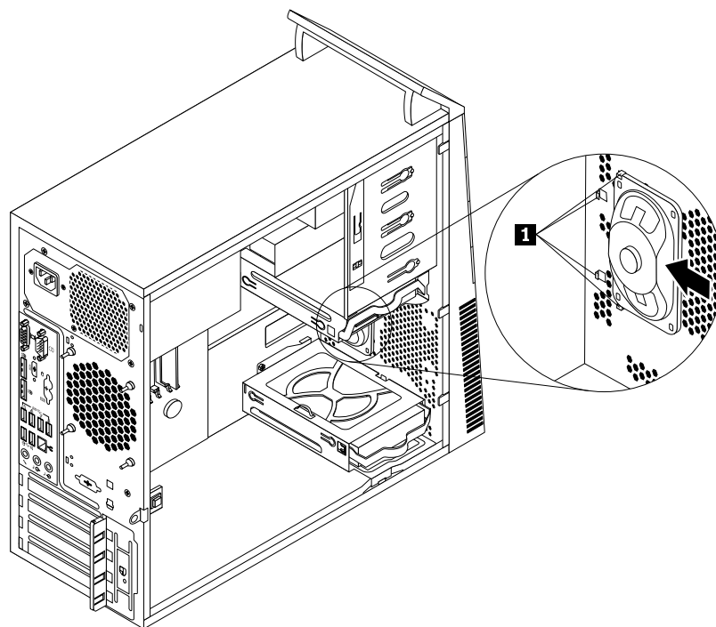
Рис. 70. Установка внутреннего динамика
