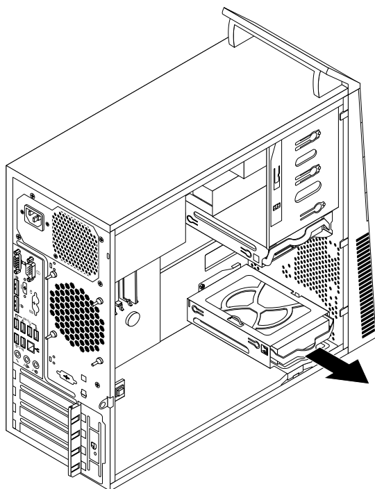
Рис. 57. Снятие дополнительного жесткого диска
