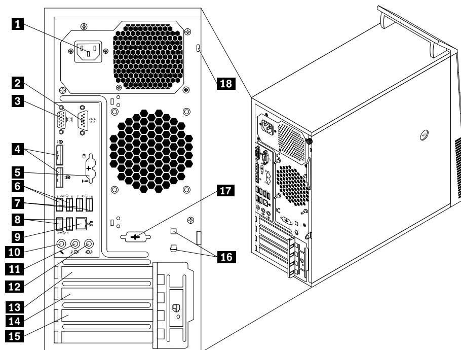
Рис. 3. Расположение разъемов на задней панели компьютера ThinkCentre M83
