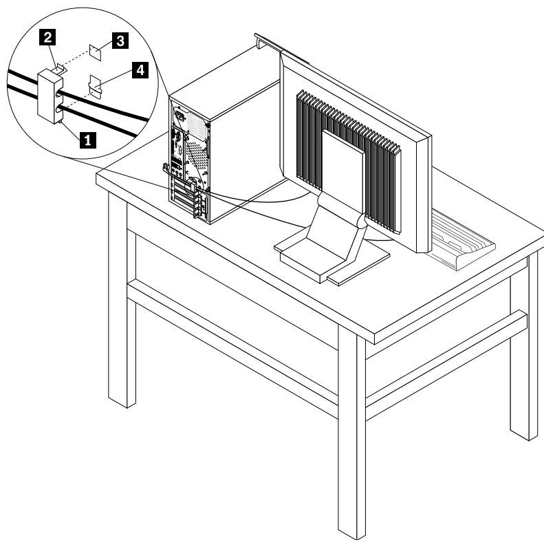
Рис. 11. Прикрепление замка для троса
