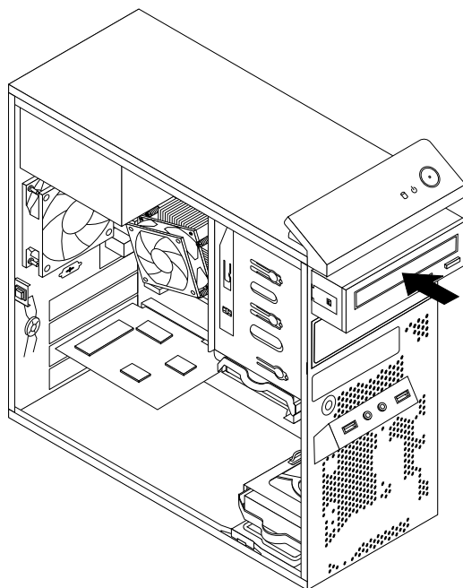
Рис. 22. Установка дисководов для оптических дисков
