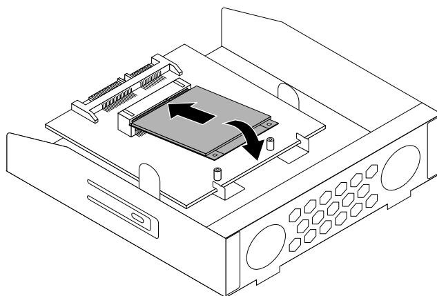
Рис. 45. Установка твердотельного диска mSATA в адаптер
