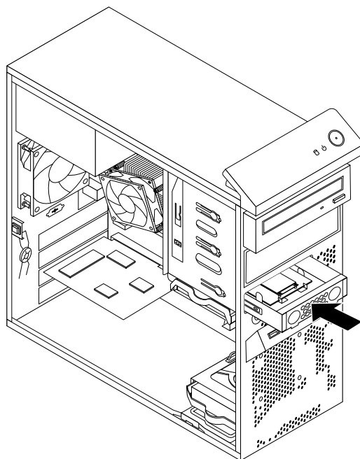
Рис. 47. Установка твердотельного диска mSATA
