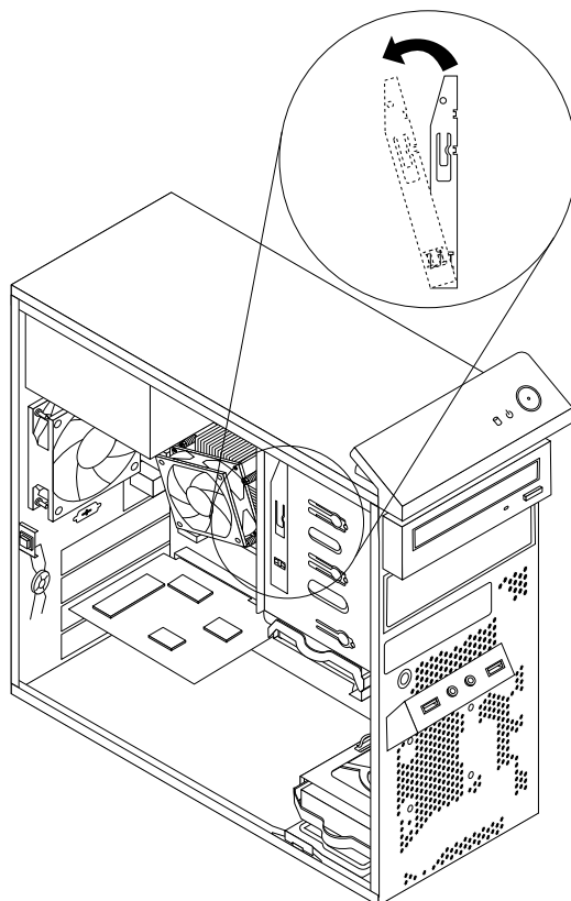
Рис. 31. Снятие крепежной скобы считывателя карт
