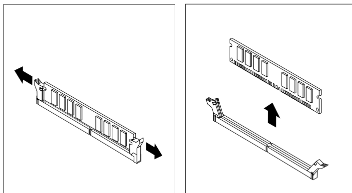
Рис. 17. Снятие модуля памяти
