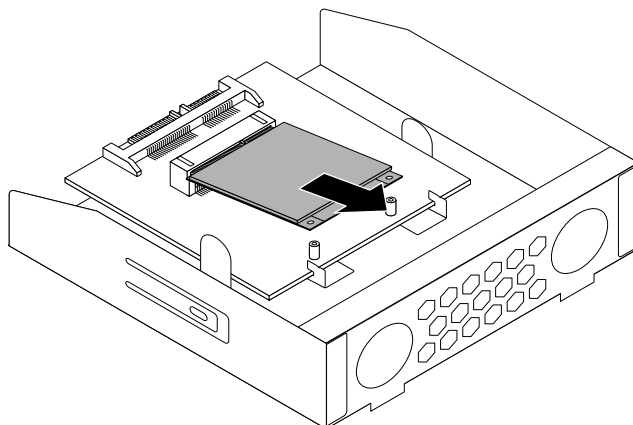
Рис. 50. Извлечение твердотельного диска mSATA
