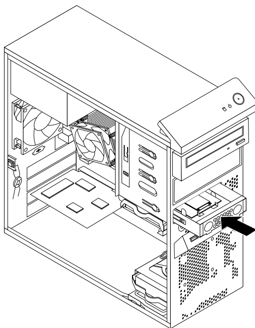
Рис. 53. Установка твердотельного диска mSATA
