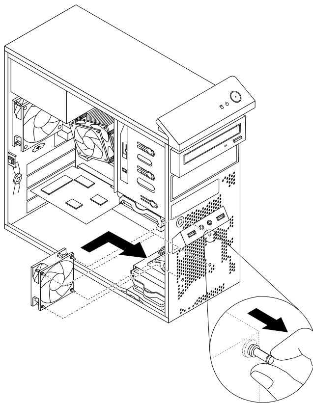
Рис. 63. Установка переднего вентилятора
