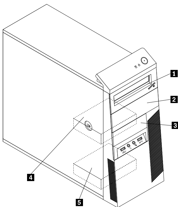
Рис. 7. Расположение отсеков для дисководов
