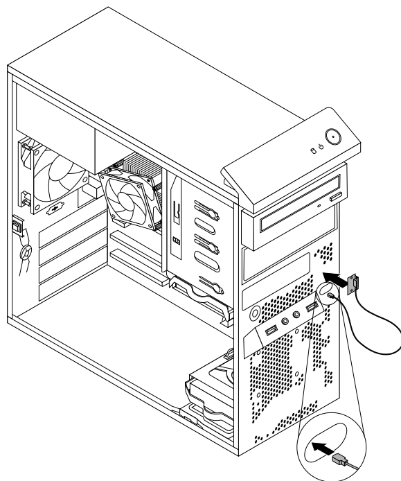
Рис. 88. Установка передней антенны Wi-Fi
