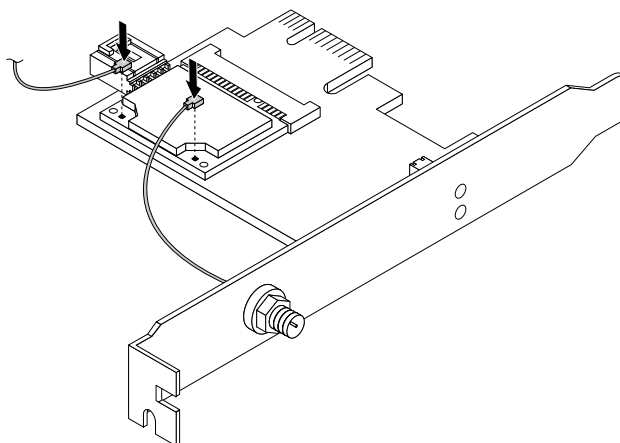
Рис. 83. Установка кабелей антенн Wi-Fi
