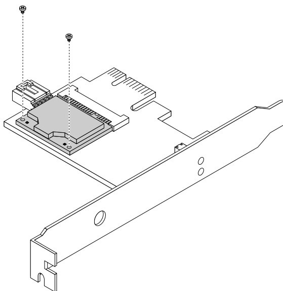
Рис. 82. Затягивание винтов для крепления модуля карты Wi-Fi
