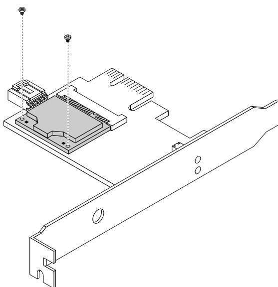
Рис. 79. Снятие винтов для крепления модуля карты Wi-Fi
