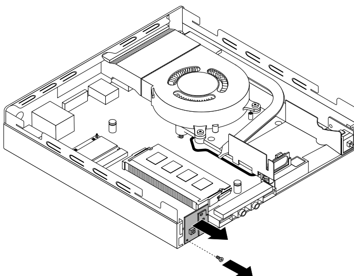
Figura 47. Rimozione della scheda dell'interruttore di alimentazione
