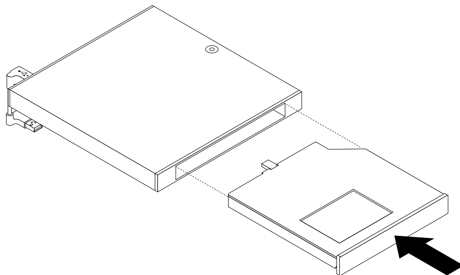
Figura 30. Installazione della staffa dell'adattatore nella scatola dell'unità ottica
