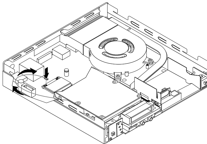
Figura 56. Collegamento del cavo dell'antenna Wi-Fi anteriore
