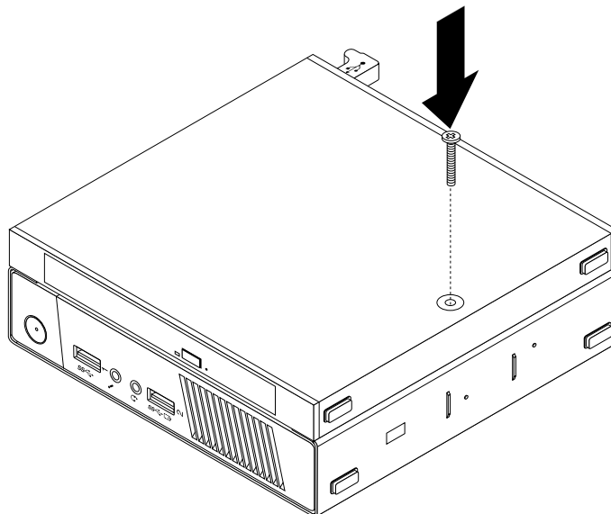
Figura 22. Installazione della vite che fissa la scatola dell'unità ottica
