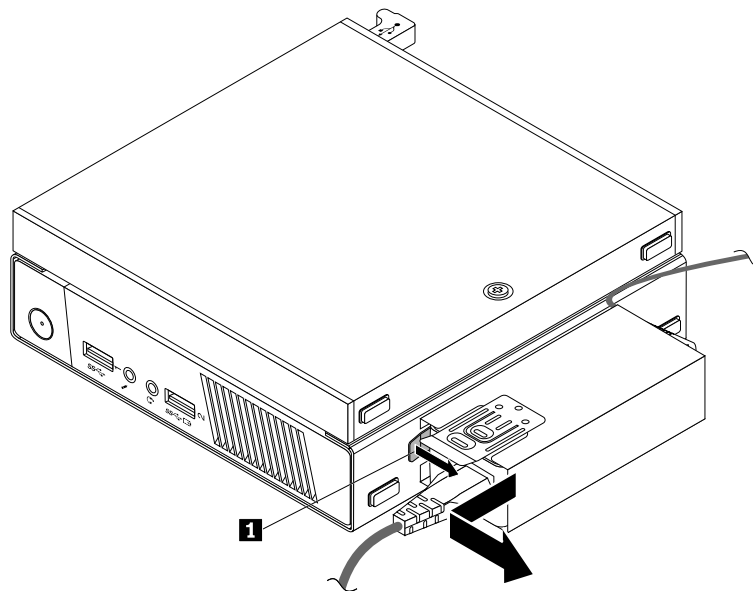
Figura 36. Rimozione della staffa dell'adattatore di alimentazione CA
