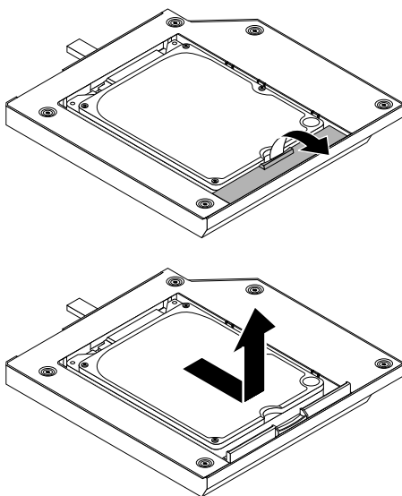
Figura 26. Rimozione dell'unità disco fisso secondaria dall'adattatore
