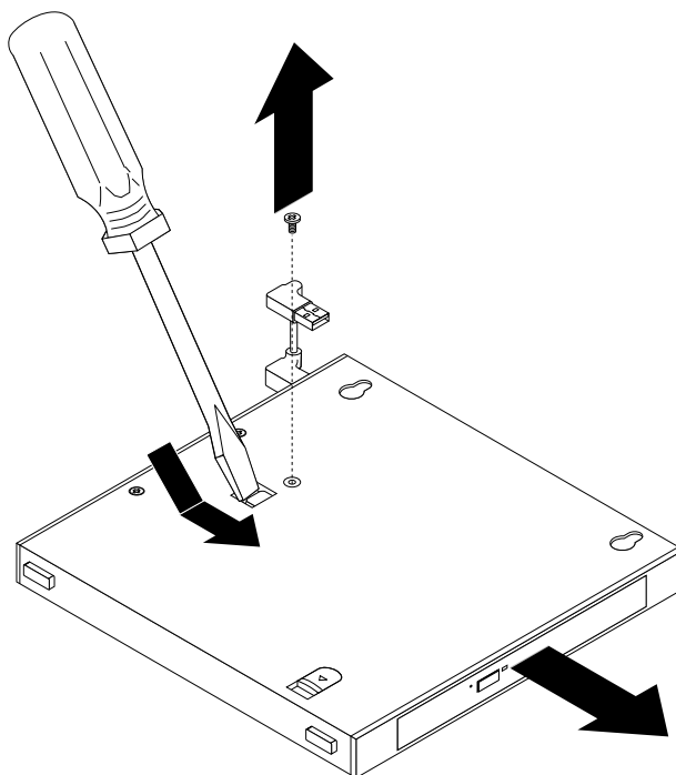
Figura 16. Rimozione dell'unità ottica dalla relativa scatola
