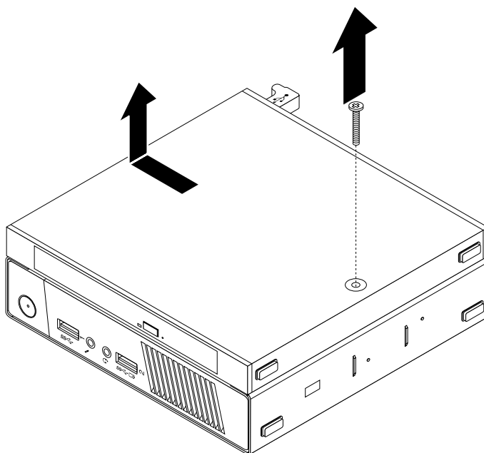
Figura 15. Rimozione della scatola dell'unità ottica
