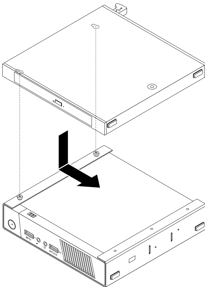
Figura 21. Installazione della scatola dell'unità ottica
