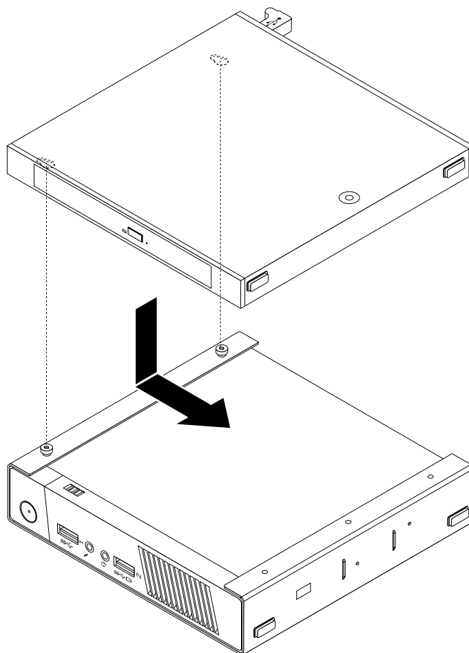
Figura 31. Installazione della scatola dell'unità ottica
