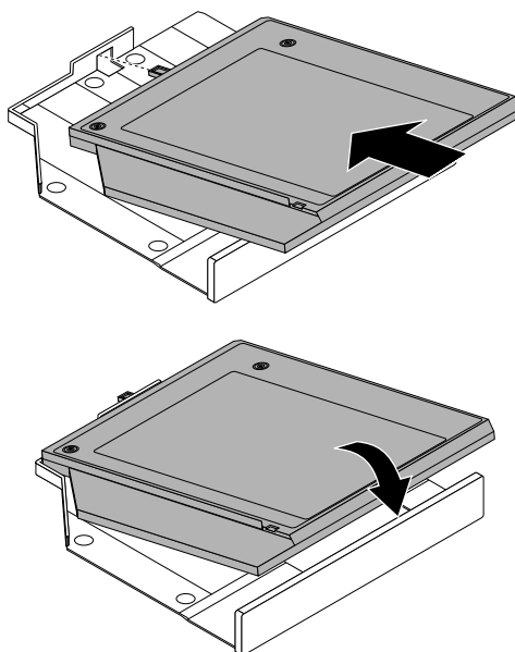
Figura 29. Installazione dell'adattatore dell'unità disco fisso nella relativa staffa
