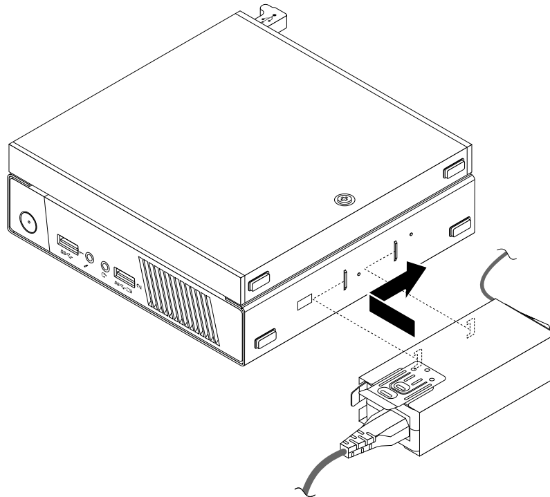
Figura 37. Installazione della staffa dell'adattatore di alimentazione CA
