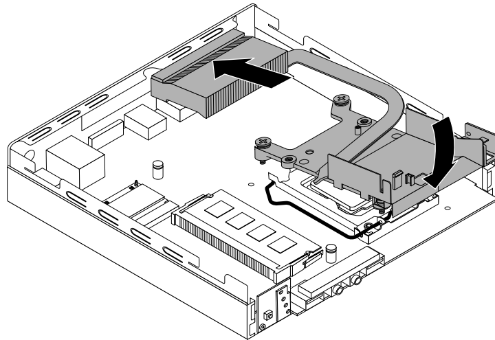
Figura 69. Installazione del modulo termico
