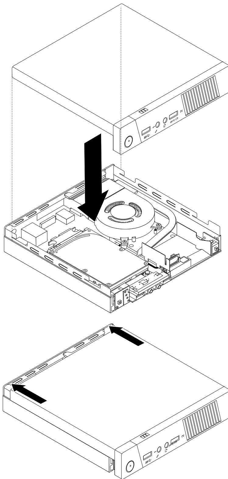
Figura 74. Installazione del coperchio del computer
