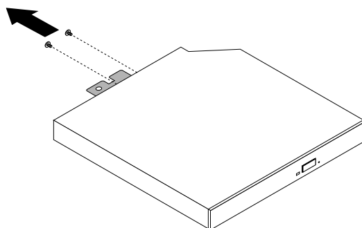
Figura 17. Rimozione della piastra di metallo dell'unità ottica
