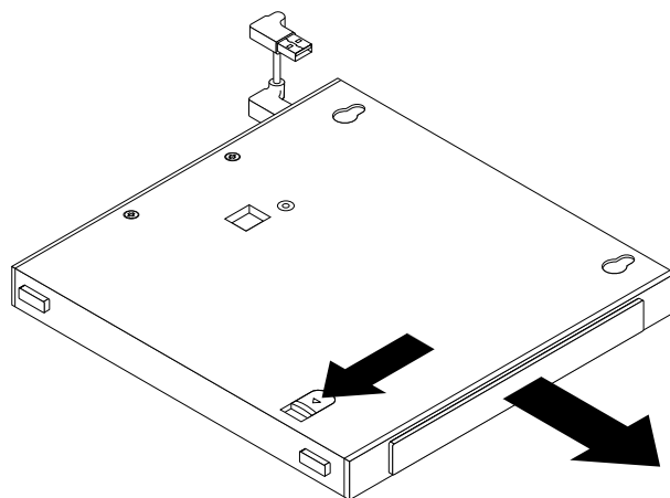
Figura 24. Rimozione dell'adattatore dell'unità disco fisso secondaria dalla scatola dell'unità ottica
