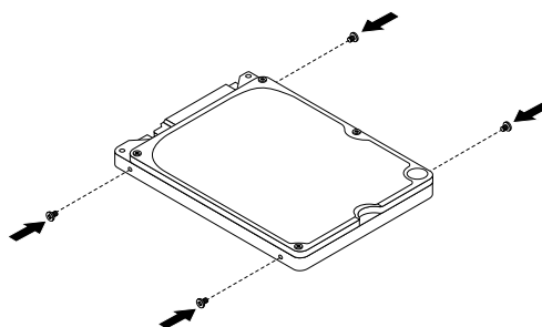
Figura 27. Installazione delle quattro viti nell'unità disco fisso
