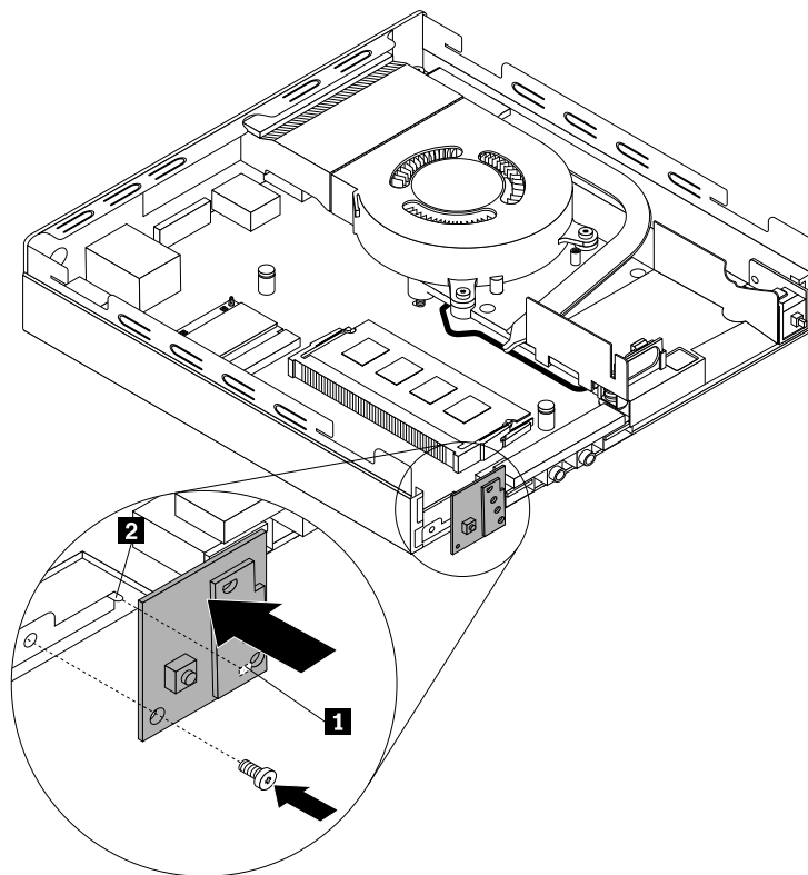
Figura 48. Installazione della scheda dell'interruttore di alimentazione
