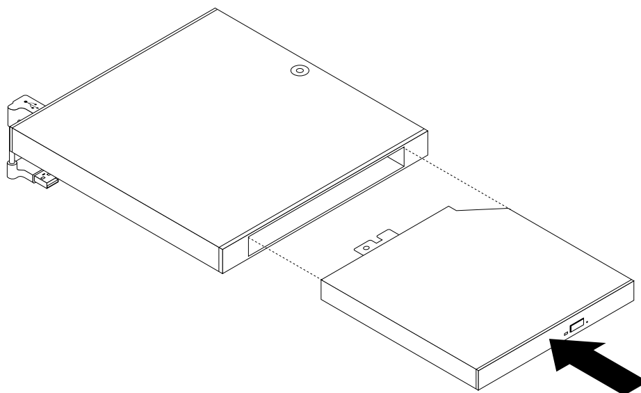
Figura 19. Installazione dell'unità ottica nella relativa scatola
