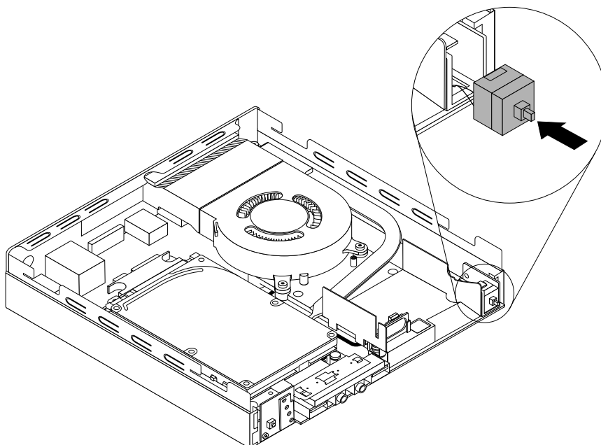
Figura 65. Installazione dell'interruttore di presenza sul coperchio
