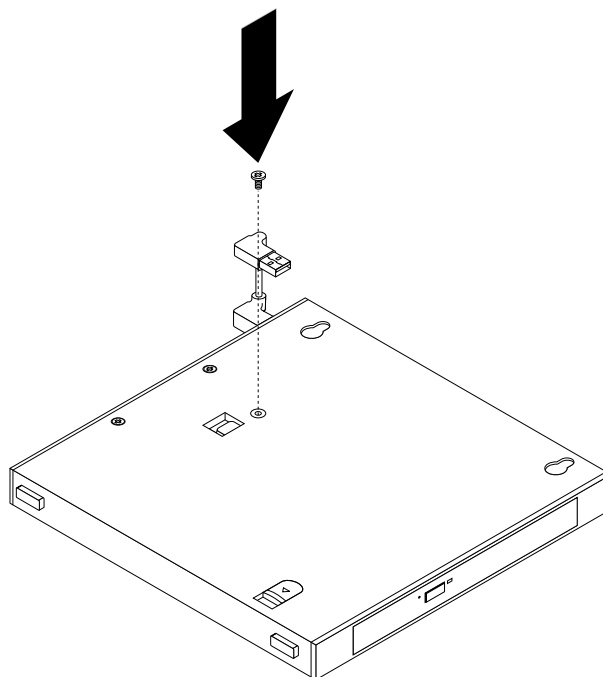
Figura 20. Installazione della vite che fissa l'unità ottica
