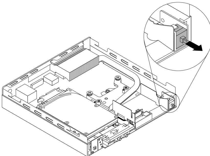
Figura 64. Rimozione dell'interruttore di presenza sul coperchio
