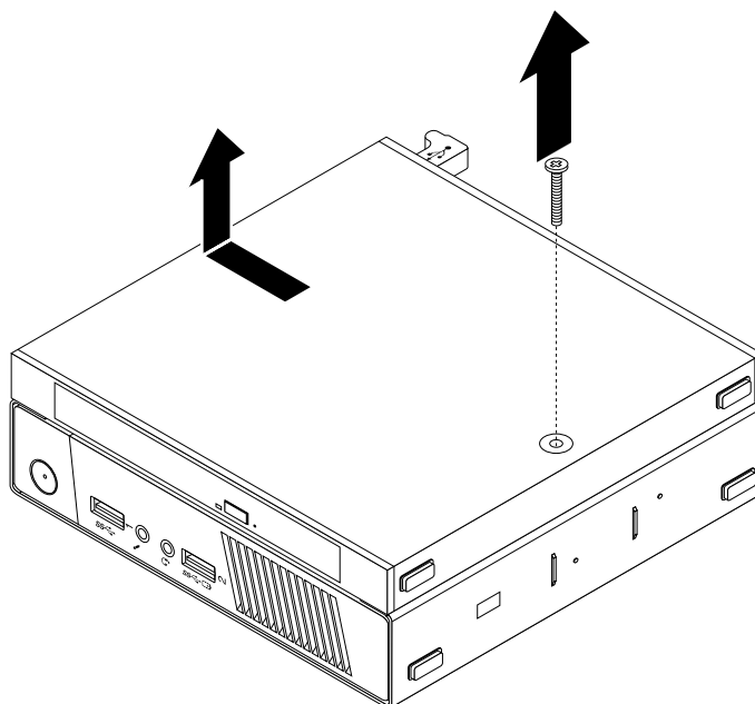
Figura 23. Rimozione della scatola dell'unità ottica
