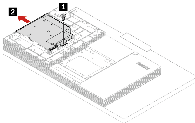
Figura 13. Extracción de la unidad óptica
