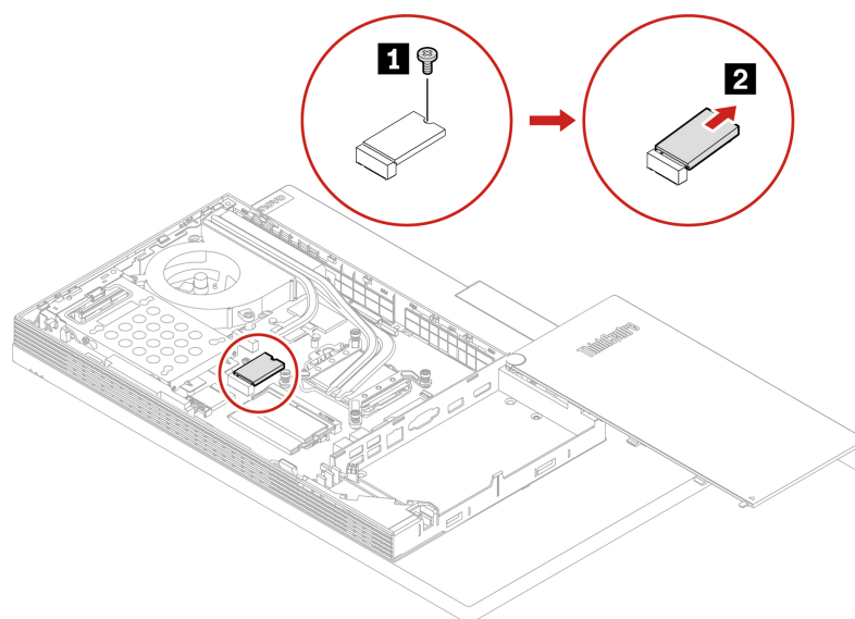
Figura 54. Extracción de la unidad de estado sólido M.2
