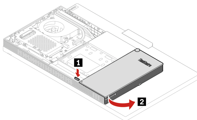
Figura 33. Apertura de la cubierta del cable
