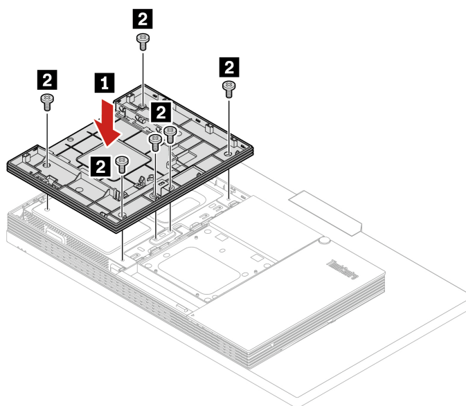
Figura 22. Instalación del soporte de la unidad óptica
