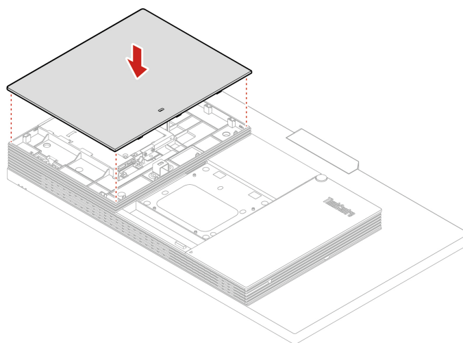
Figura 12. Instalación de la cubierta posterior
