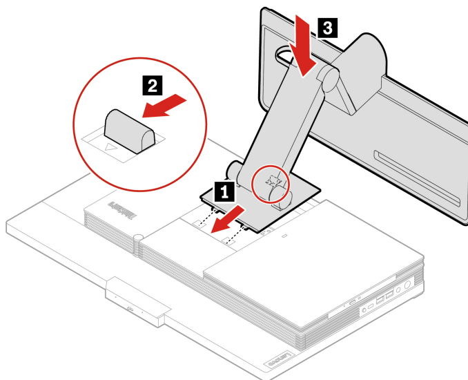
Figura 10. Instalar el pedestal UltraFlex IV
