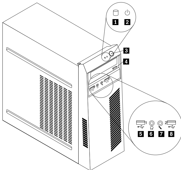
Figura 1. Posições dos conectores, controles e indicadores frontais
