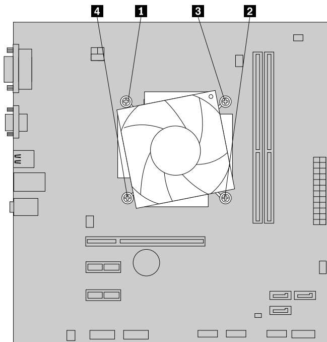
Figura 27. Removendo o Conjunto do Dissipador de Calor e do Ventilador
