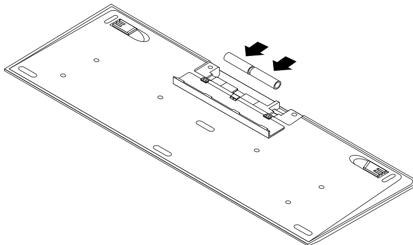
Figura 11. Instalar as pilhas do teclado
