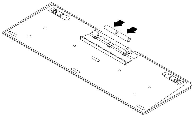
図11. キーボード・バッテリーの取り付け
