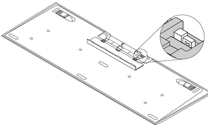
図 13. キーボードのバッテリー・コンパートメントへのdongleの保管
