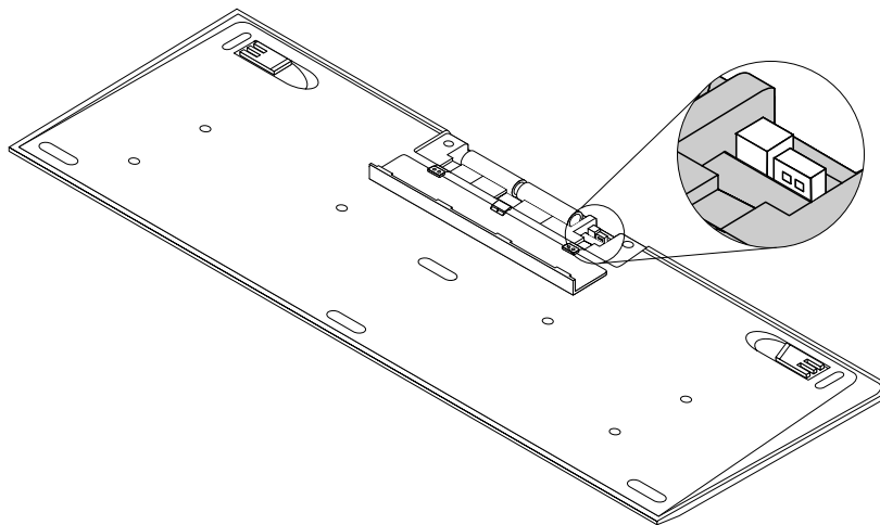
Figura 13. Almacenamiento de la mochila en el compartimiento de la batería del teclado.
