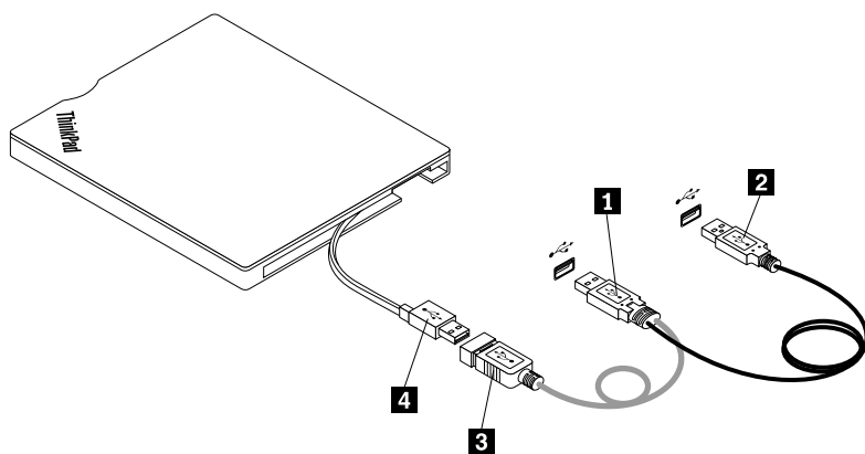
图 2. 连接驱动器
