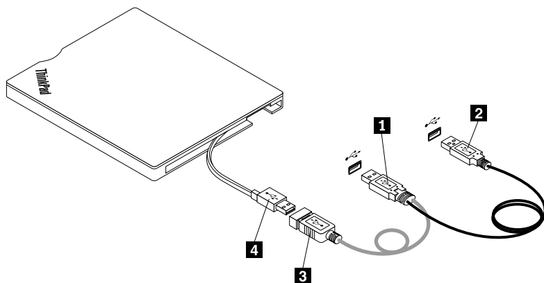
Рис. 2. Подключение дисковода
