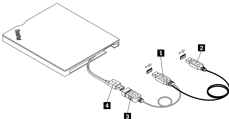
Figura 2. Connessione dell'unità
