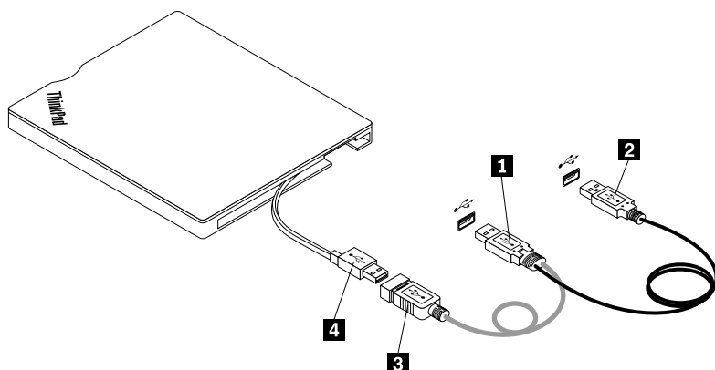
Obrázek 2. Připojení jednotky
