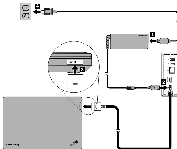
Rysunek 3. Podłączanie stacji dokującej do gniazda zasilającego i notebooka
