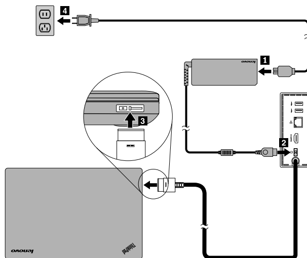
Figura 3. Collegamento del dock all'alimentatore e al computer notebook
