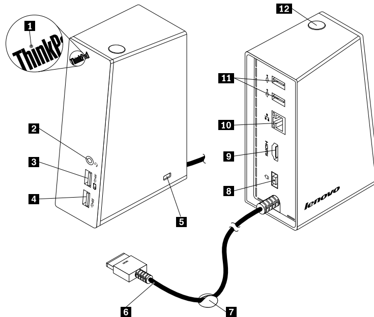
Figura 1. Visión general de la estación de acoplamiento
