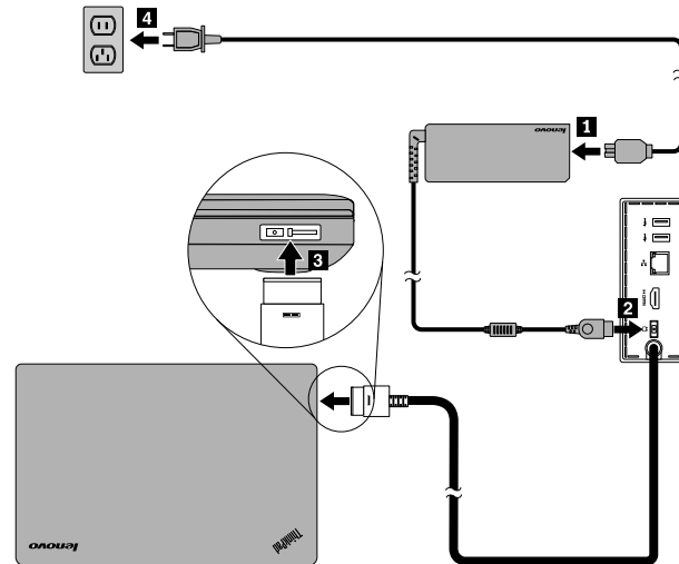
Abbildung 3. Andockstation an Netzteil und Ihren Notebook-Computer anschließen
