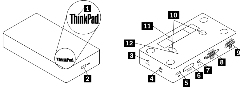
Şekil1. Kablosuz ekran bađdařtırıcısına genel bakıř
