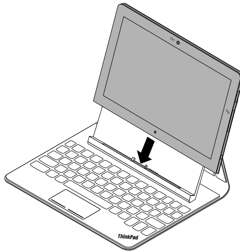
Figura 3. Allineare il connettore per tastiera sul tablet con il connettore per tastiera sul touch case
