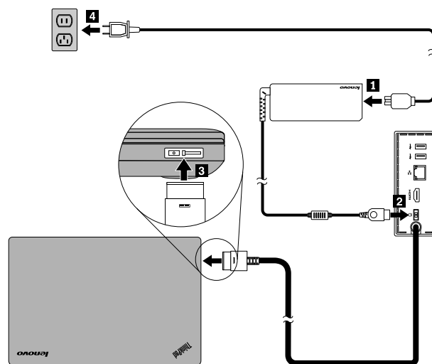
Figura 3. Conectando o dock à fonte de alimentação e ao computador notebook
