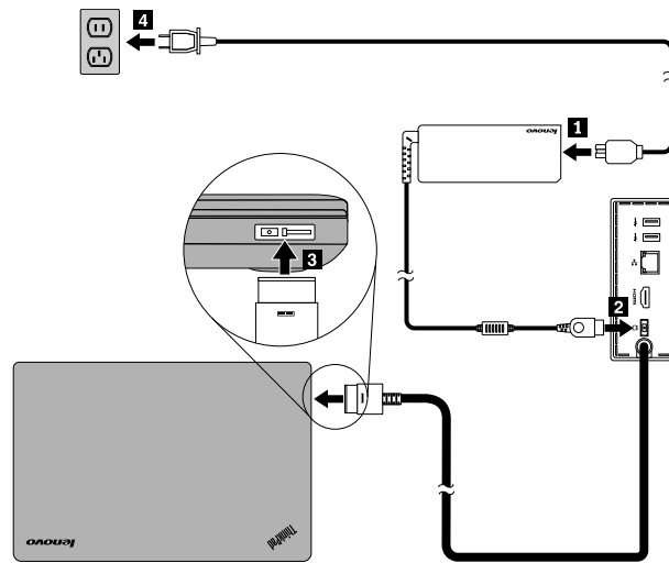
Figura 3. Conexión de la estación de acoplamiento a la fuente de alimentación y al sistema portátil
