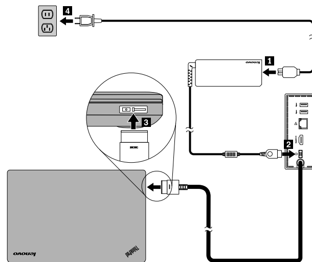
Abbildung 3. Andockstation an Netzteil und Ihren Notebook-Computer anschließen
