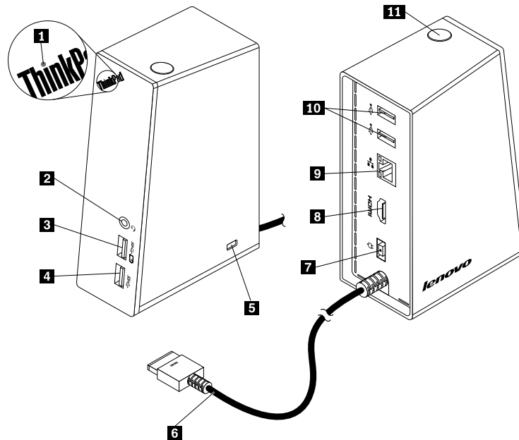
Abbildung 1. Andockstation – Übersicht
