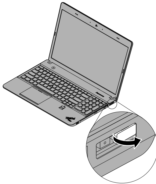
Abbildung 2. Lenovo OneLink-Steckplatzabdeckung entfernen
