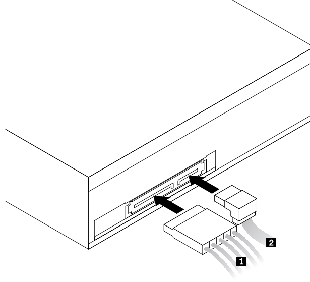
Şekil1. Güç kablosunun ve SATA kablosunun sürücünün arkasına bağlanması
