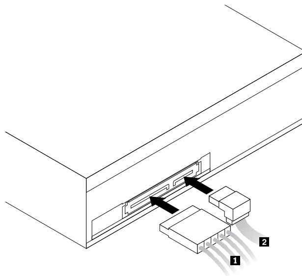
Obrázok 1. Pripojenie napájacieho kábla a kábla SATA k zadnej strane jednotky
