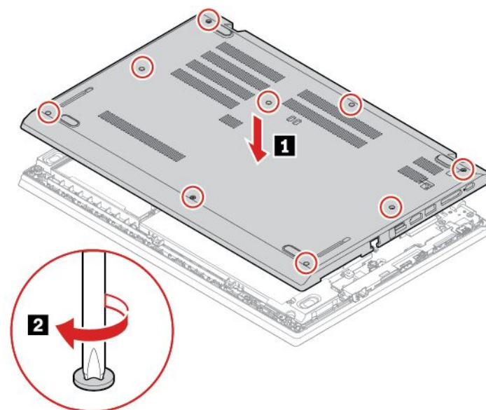
図 7. L590 のベース・カバー・アセンブリーの取り付け
