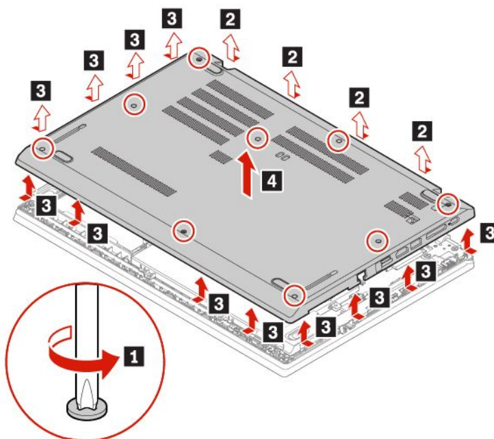
図 5. L590 のベース・カバー・アセンブリーの取り外し
