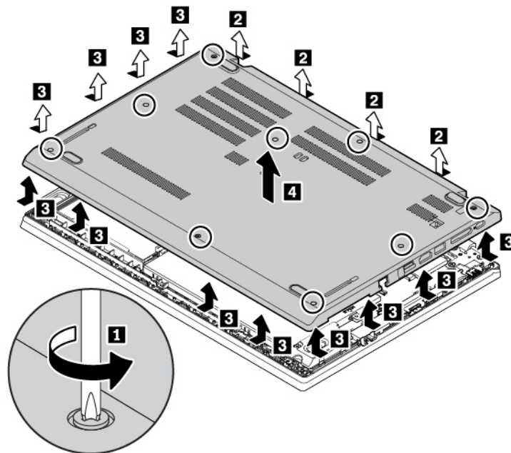
Figuur 5. De klep aan de onderkant van de computer verwijderen voor ThinkPad L580-computers
