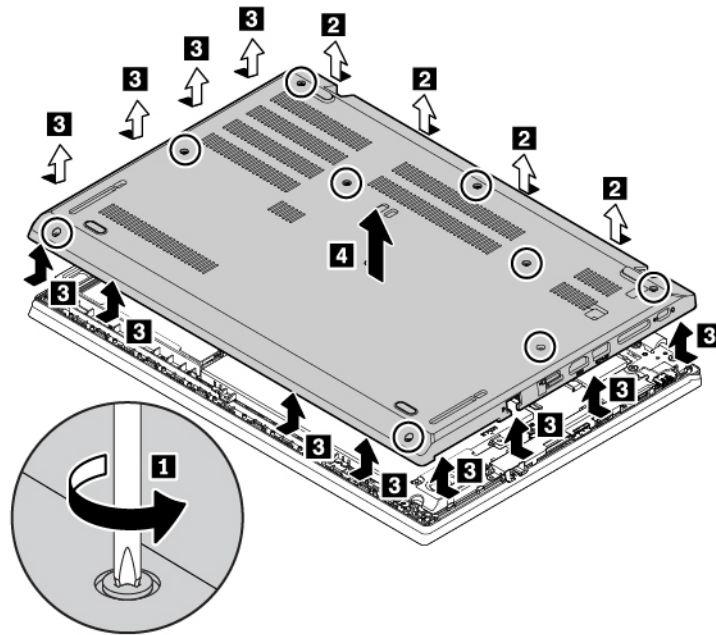
Figuur 4. De klep aan de onderkant van de computer verwijderen voor ThinkPad L480-computers
