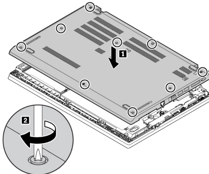
Figuur 7. De klep aan de onderkant van de computer installeren voor ThinkPad L580-computers
