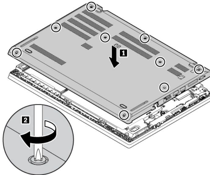
Figuur 6. De klep aan de onderkant van de computer installeren voor ThinkPad L480-computers
