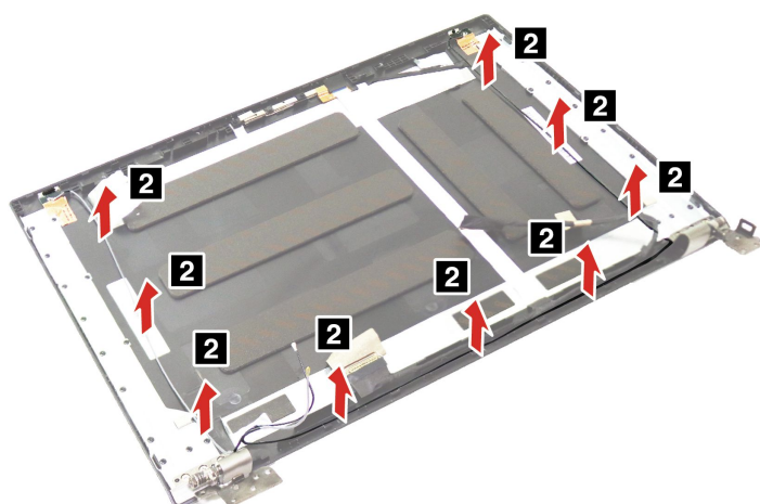
ワイヤレス WAN アンテナ (一部のモデル向け) の取り外し手順
