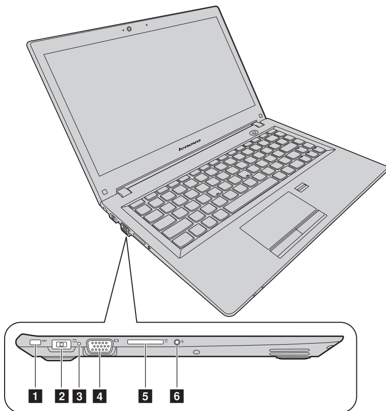
圖 2. 左側視圖
