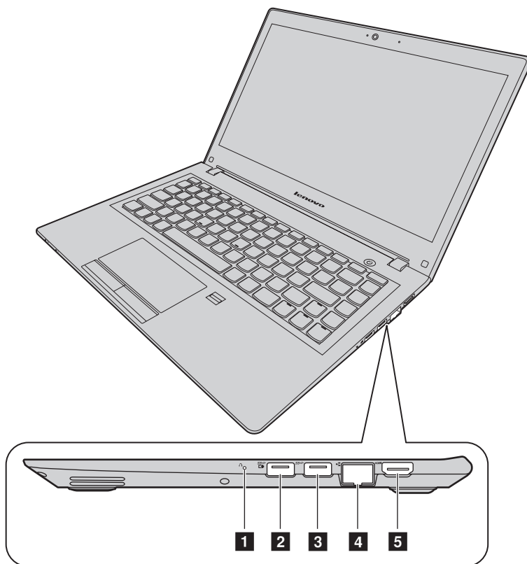
圖 3. 右側視圖
