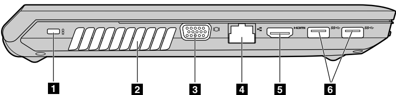
Рис. 2. Lenovo B480 и B580 (вид слева)
