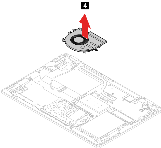
Figure 34. Remove the fan
